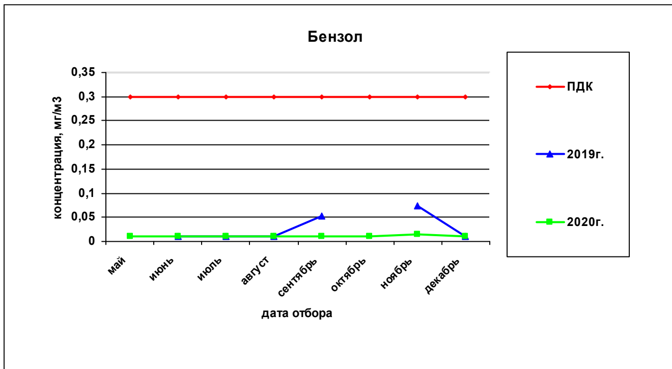
Рисунок 61— Сравнительная характеристика изменения концентрации бензола в атмосферном воздухе у домов по ул. Вавилова, 21 – Малкова, 22 за 2019 и 2020гг.
