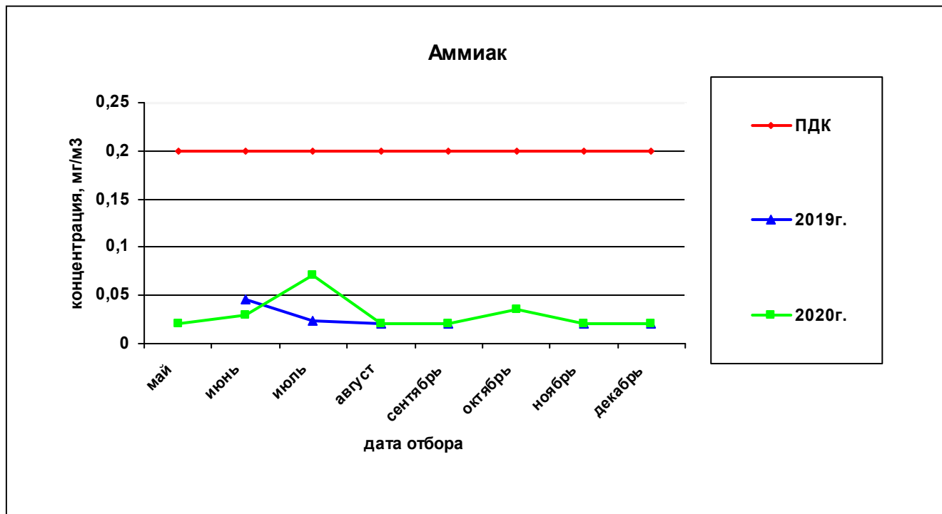
Рисунок 70— Сравнительная характеристика изменения концентрации аммиака в атмосферном воздухе на ул.Петропавловская,185 за 2019 и 2020гг.
