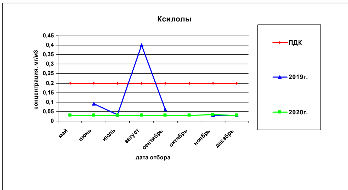
Рисунок 63— Сравнительная характеристика изменения концентрации КСИЛОЛОВ в атмосферном воздухе у домов по ул. Вавилова, 21 – Малкова, 22 за 2019 и 2020гг.
