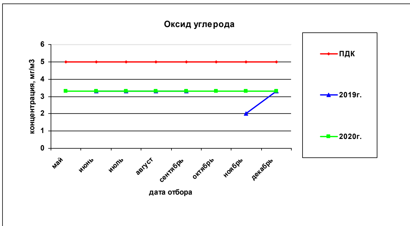
Рисунок 55— Сравнительная характеристика изменения концентрации оксида углерода в атмосферном воздухе у домов по ул. Вавилова, 21 – Малкова, 22 за 2019 и 2020гг.
