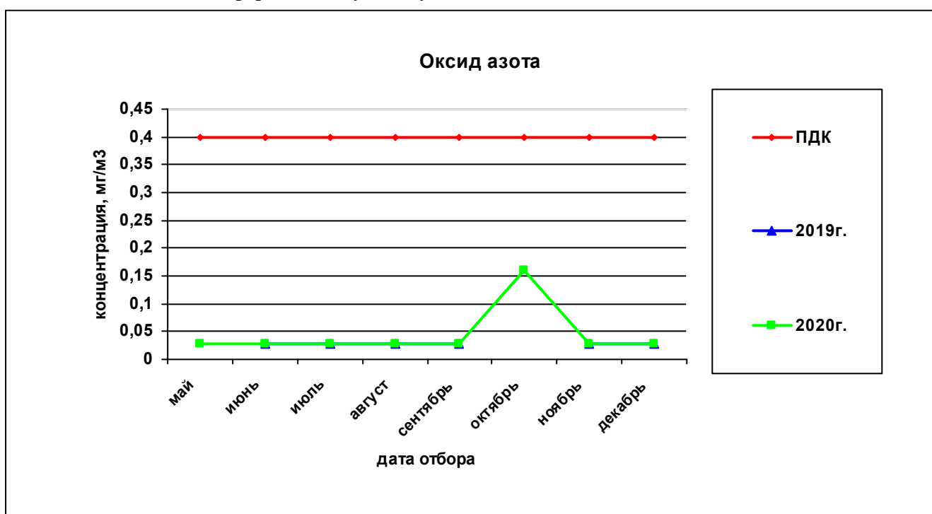
Рисунок 18— Сравнительная характеристика изменения концентрации оксида азота в атмосферном воздухе на ул. Костычева за 2019 и 2020гг.
