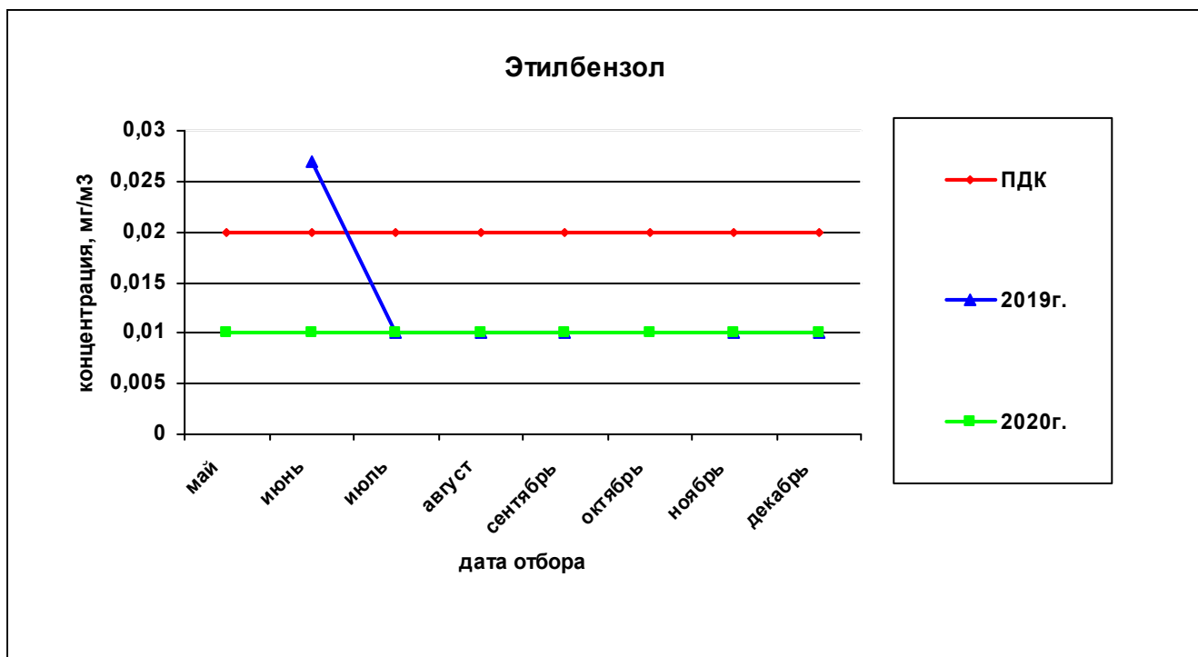
Рисунок 48— Сравнительная характеристика изменения концентрации ЭТИЛБЕНЗОЛА в атмосферном воздухе на ул. Строителей, 16 за 2019 и 2020гг.
