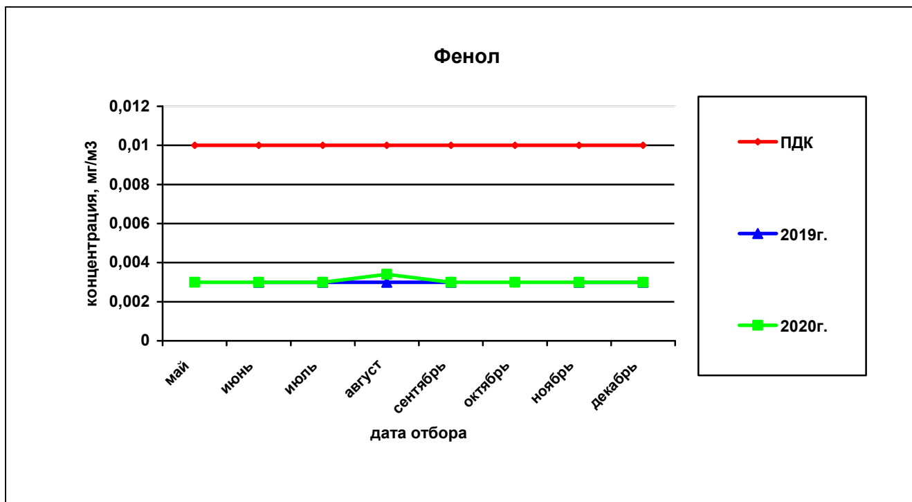
Рисунок 72— Сравнительная характеристика изменения концентрации фенола в атмосферном воздухе на ул.Петропавловская,185 за 2019 и 2020гг.
