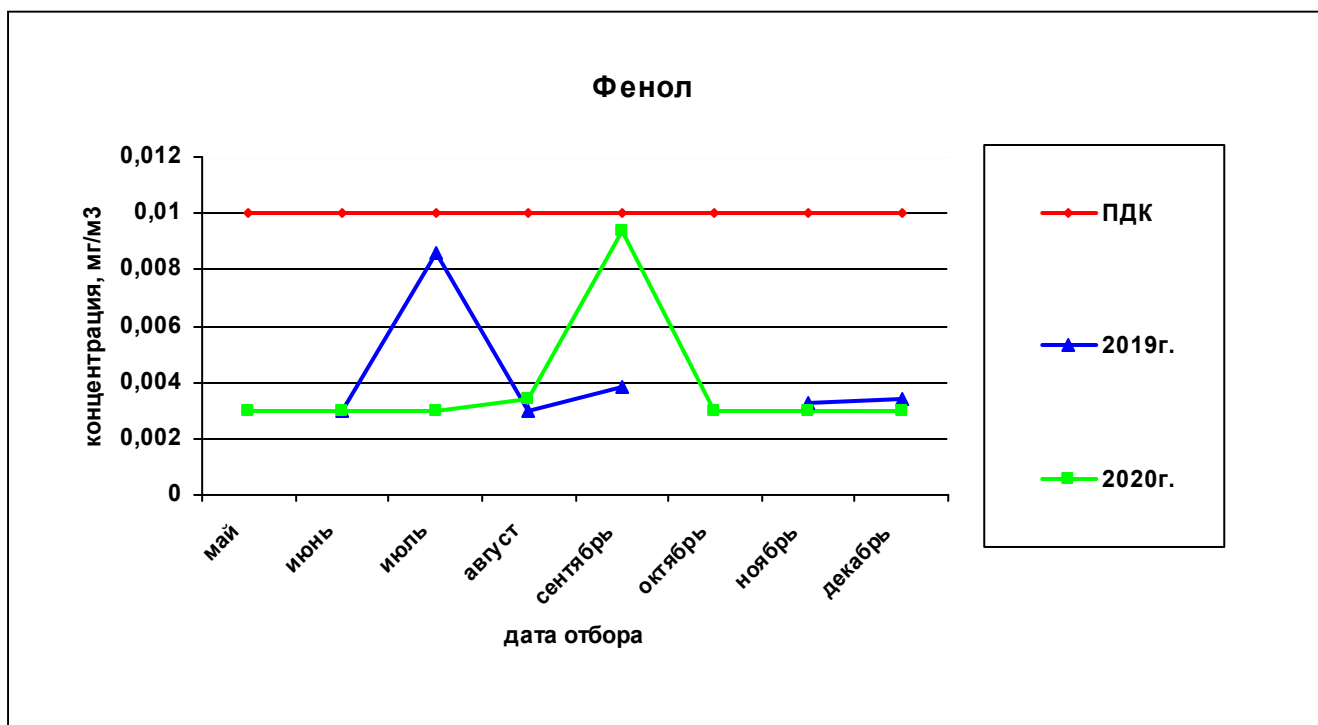
Рисунок 24— Сравнительная характеристика изменения концентрации фенола в атмосферном воздухе на ул. Костычева за 2019 и 2020гг.
