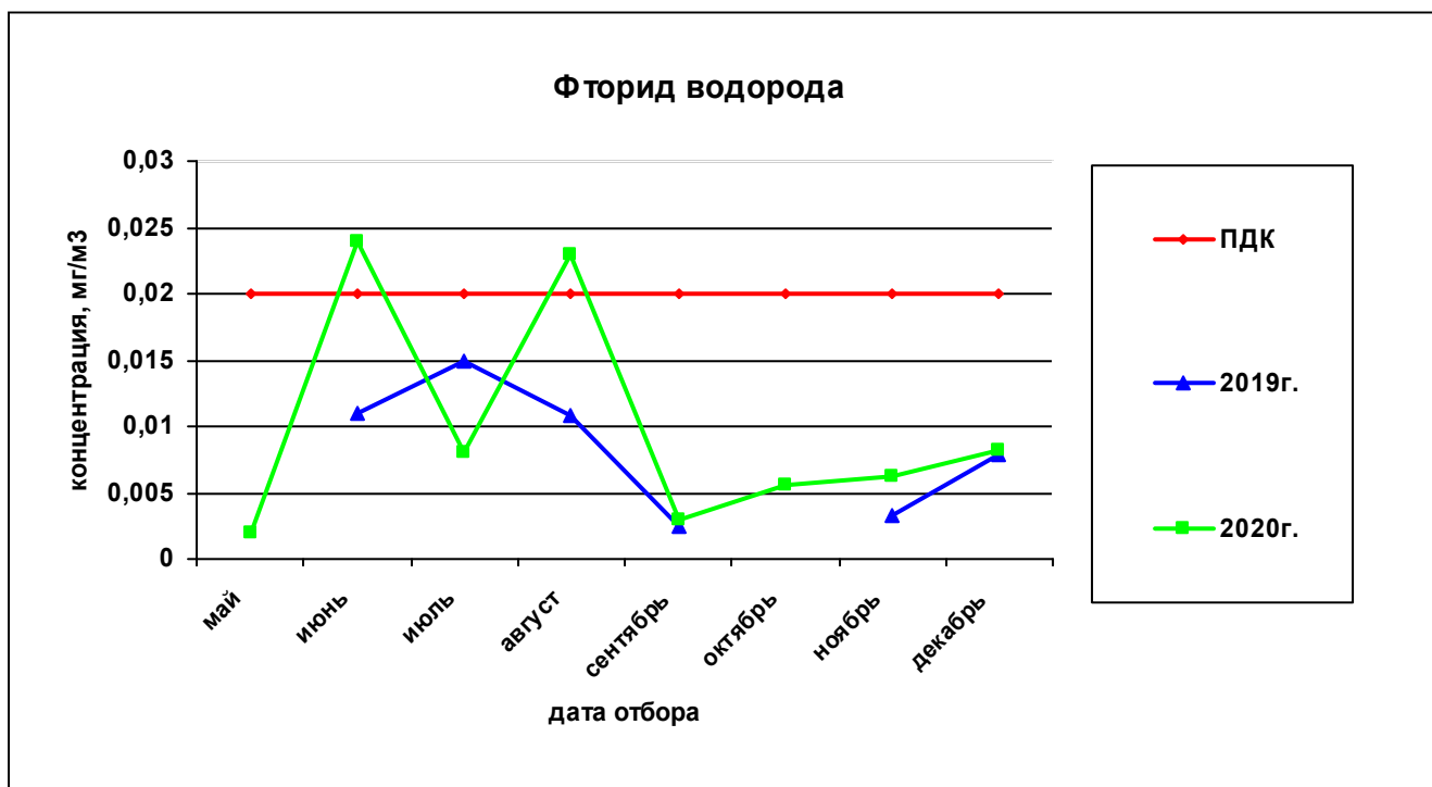
Рисунок 27— Сравнительная характеристика изменения концентрации фторида водорода в атмосферном воздухе на ул. Костычева за 2019 и 2020гг.
