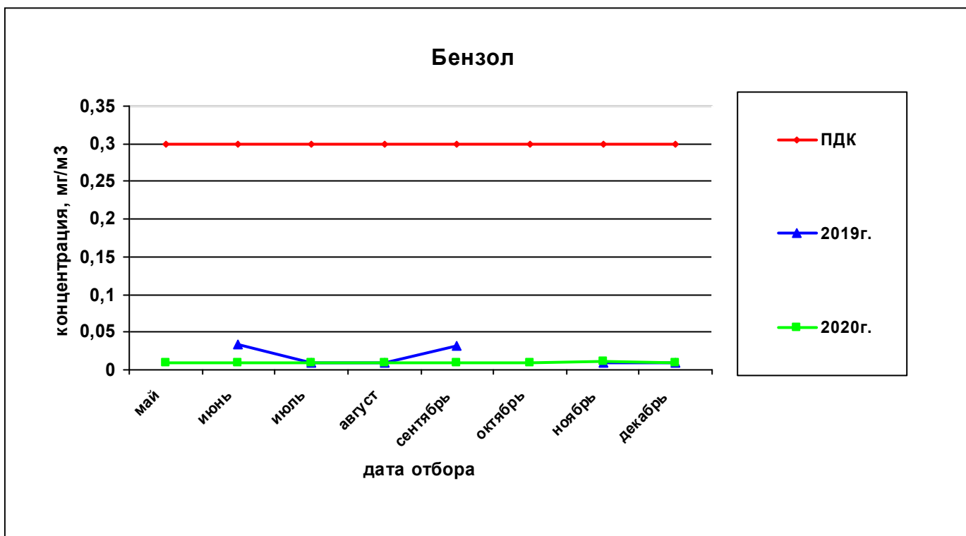
Рисунок 77— Сравнительная характеристика изменения концентрации бензола в атмосферном воздухе на ул.Петропавловская,185 за 2019 и 2020гг.
