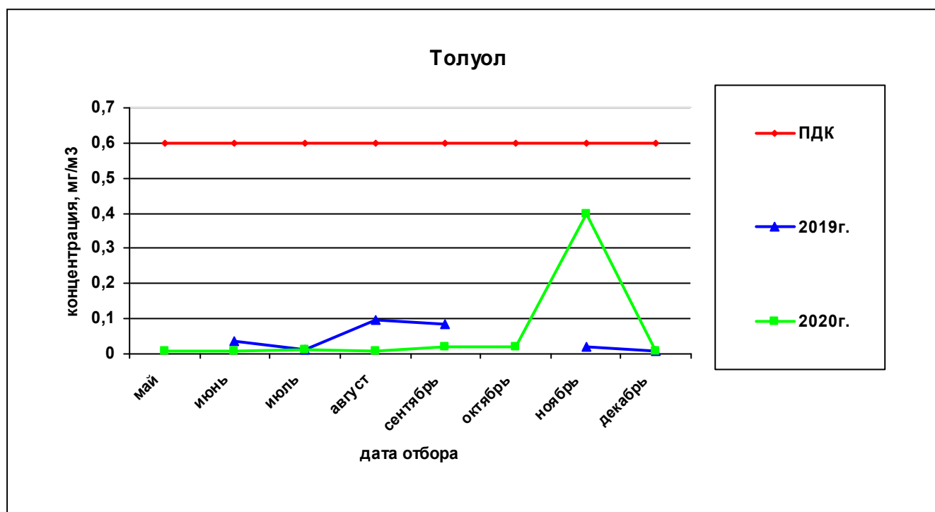
Рисунок 30— Сравнительная характеристика изменения концентрации толуола в атмосферном воздухе на ул. Костычева за 2019 и 2020гг.
