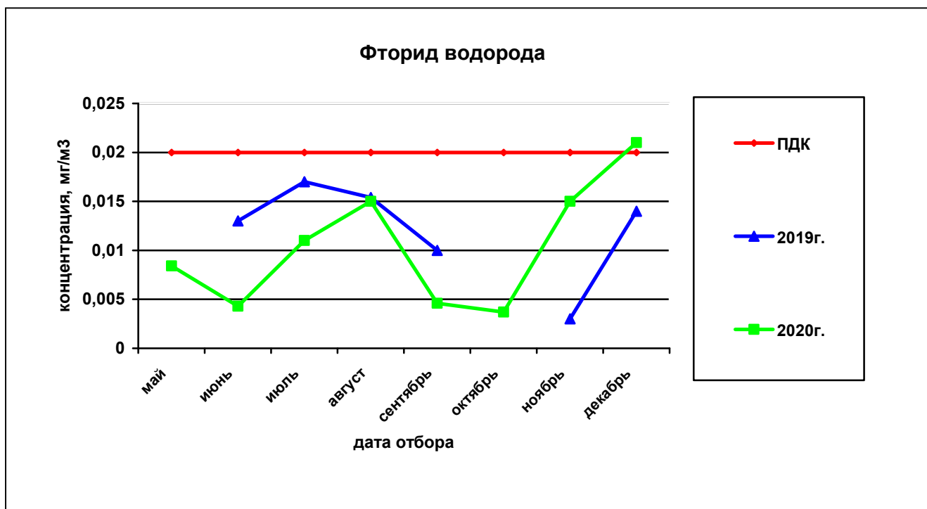
Рисунок 59— Сравнительная характеристика изменения концентрации фторида водорода в атмосферном воздухе у домов по ул. Вавилова, 21 – Малкова, 22 за 2019 и 2020гг.
