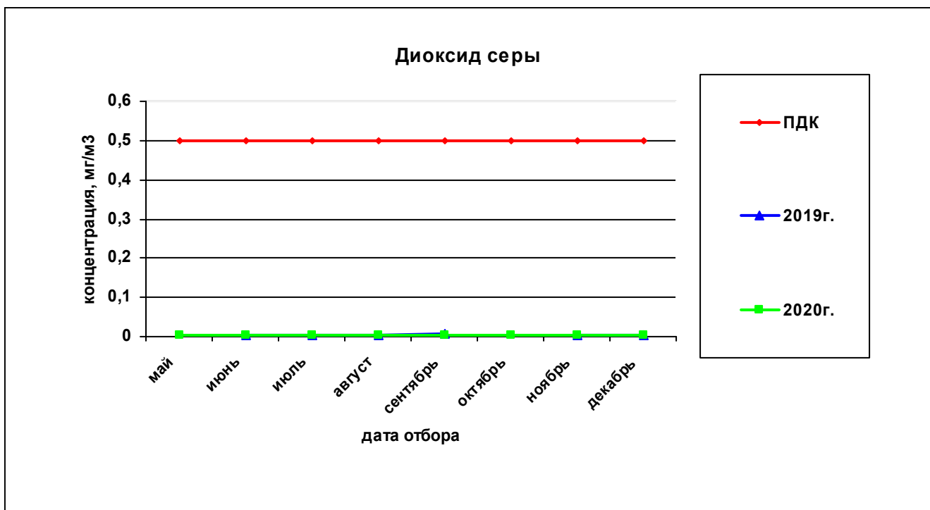
Рисунок 68— Сравнительная характеристика изменения концентрации диоксида серы в атмосферном воздухе на ул.Петропавловская,185 за 2019 и 2020гг.
