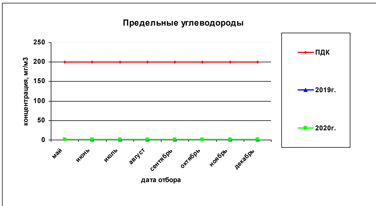
Рисунок 60— Сравнительная характеристика изменения концентрации предельных углеводородов в атмосферном воздухе у домов по ул. Вавилова, 21 – Малкова, 22 за 2019 и 2020гг.
