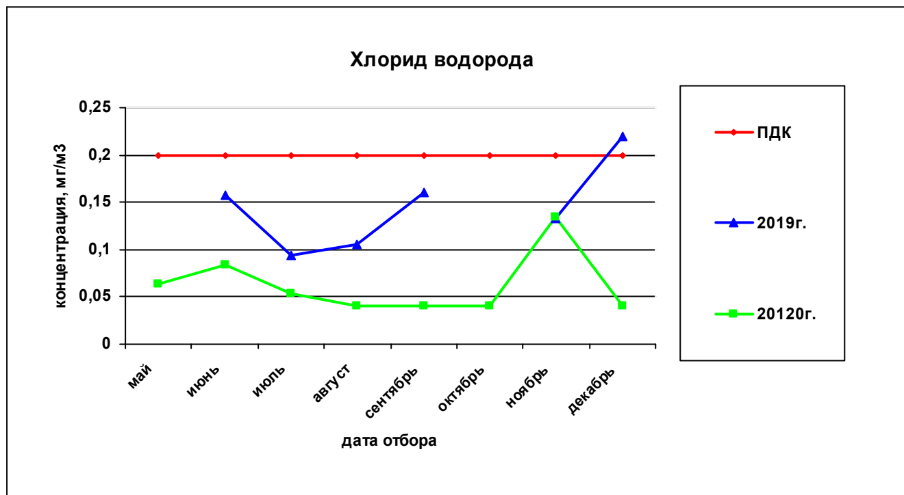
Рисунок 19— Сравнительная характеристика изменения концентрации хлорида водорода в атмосферном воздухе на ул. Костычева за 2019 и 2020гг.
