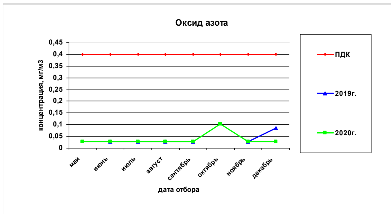
Рисунок 34— Сравнительная характеристика изменения концентрации оксида азота в атмосферном воздухе на ул. Строителей, 16 за 2019 и 2020гг.
