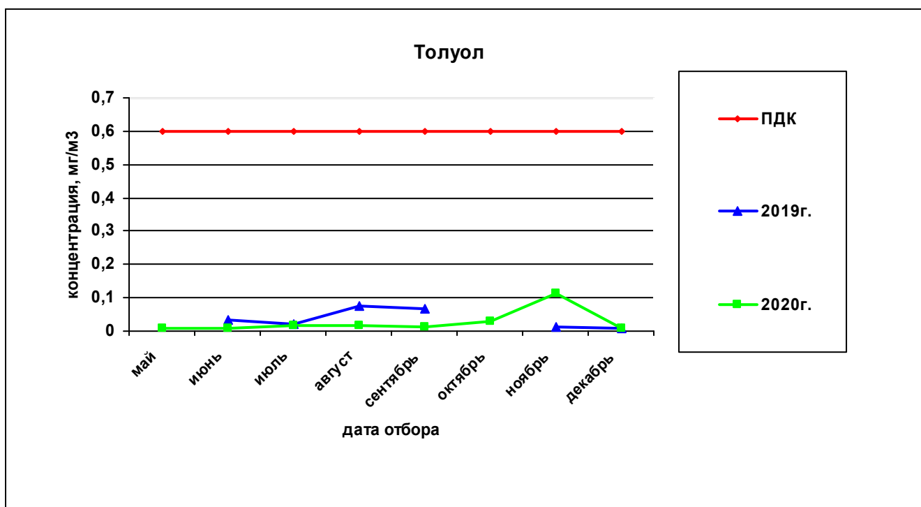
Рисунок 46— Сравнительная характеристика изменения концентрации толуола в атмосферном воздухе на ул. Строителей, 16 за 2019 и 2020гг.
