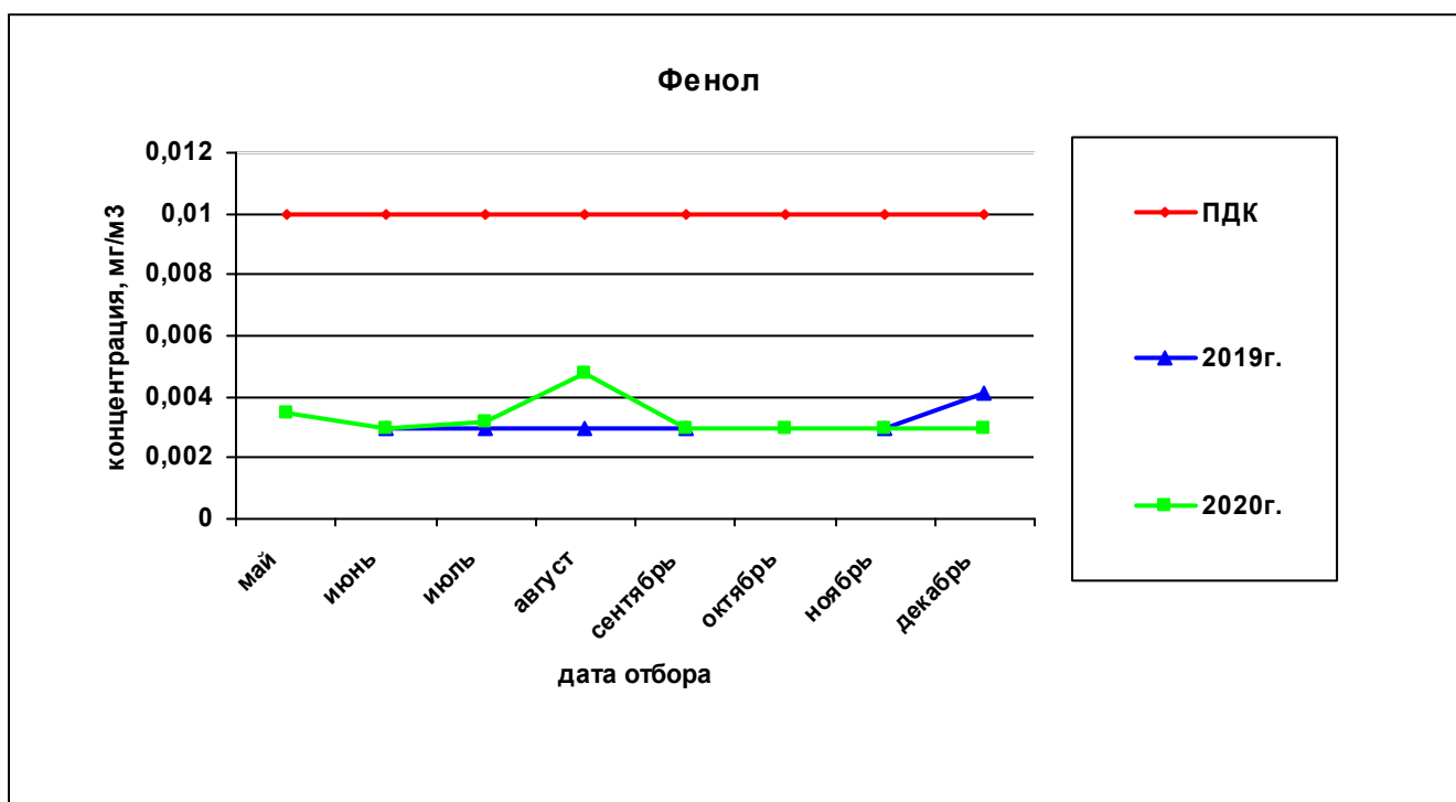
Рисунок 56— Сравнительная характеристика изменения концентрации фенола в атмосферном воздухе у домов по ул. Вавилова, 21 – Малкова, 22 за 2019 и 2020гг.
