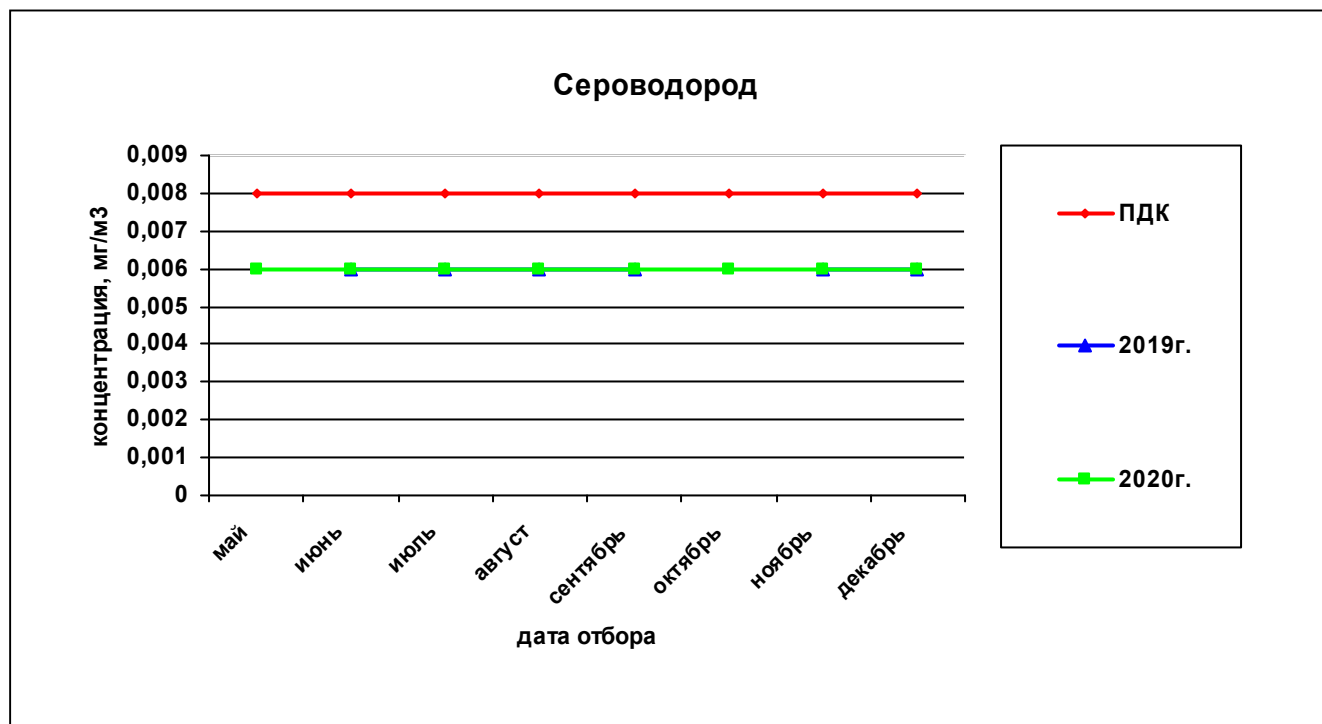
Рисунок 37— Сравнительная характеристика изменения концентрации сероводорода в атмосферном воздухе на ул. Строителей, 16 за 2019 и 2020гг.
