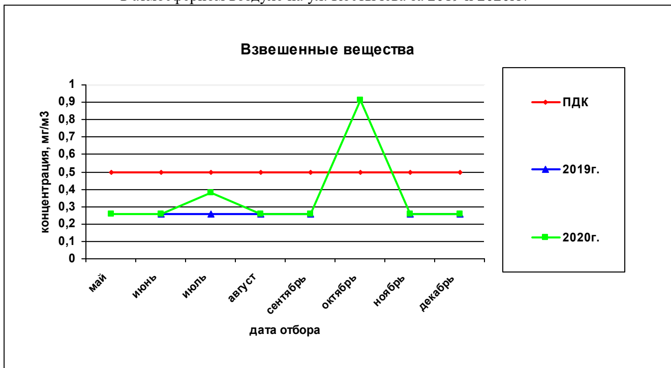
Рисунок 26— Сравнительная характеристика изменения концентрации взвешенных веществ в атмосферном воздухе на ул. Костычева за 2019 и 2020гг.
