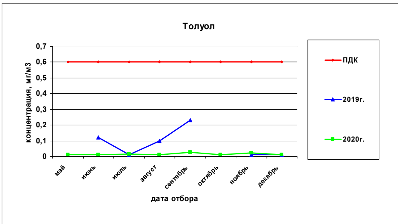
Рисунок 78— Сравнительная характеристика изменения концентрации толуола в атмосферном воздухе на ул.Петропавловская,185 за 2019 и 2020гг.
