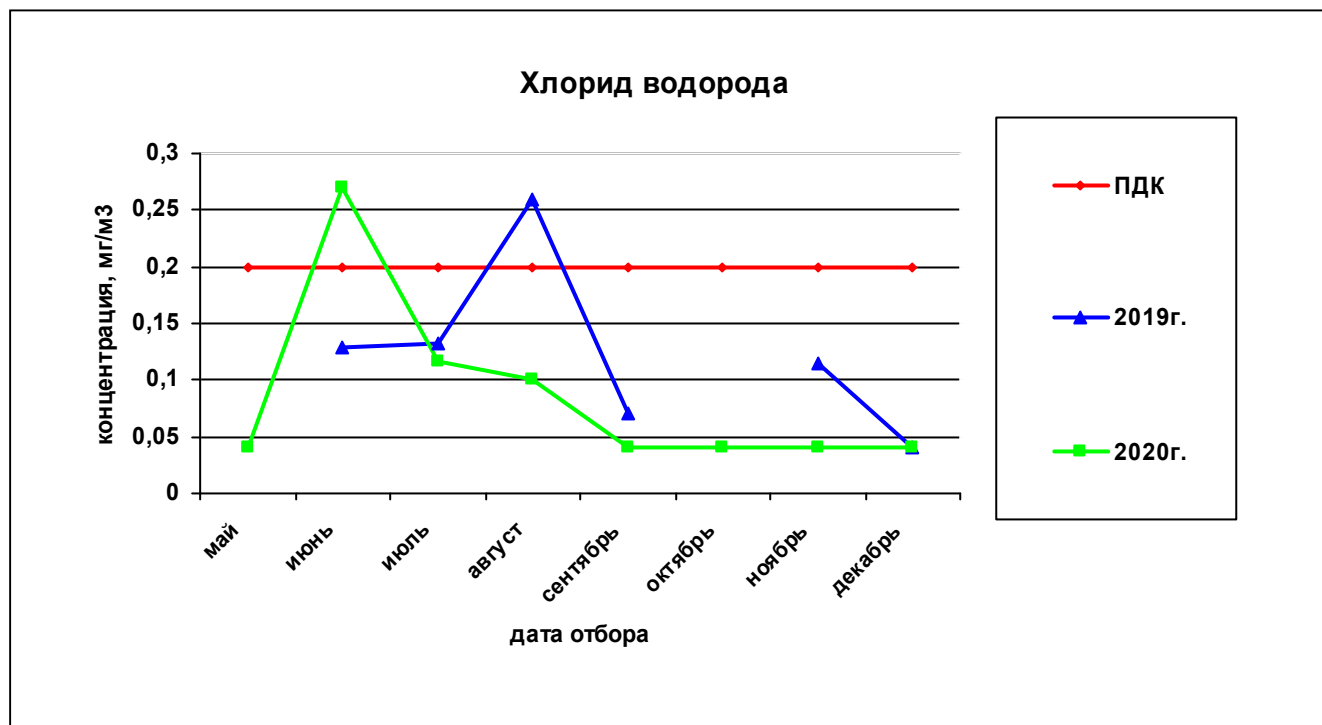
Рисунок 67— Сравнительная характеристика изменения концентрации хлорида водорода в атмосферном воздухе на ул.Петропавловская,185 за 2019 и 2020гг.
