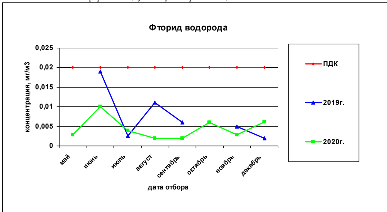
Рисунок 43— Сравнительная характеристика изменения концентрации фторида водорода в атмосферном воздухе на ул. Строителей, 16 за 2019 и 2020гг.
