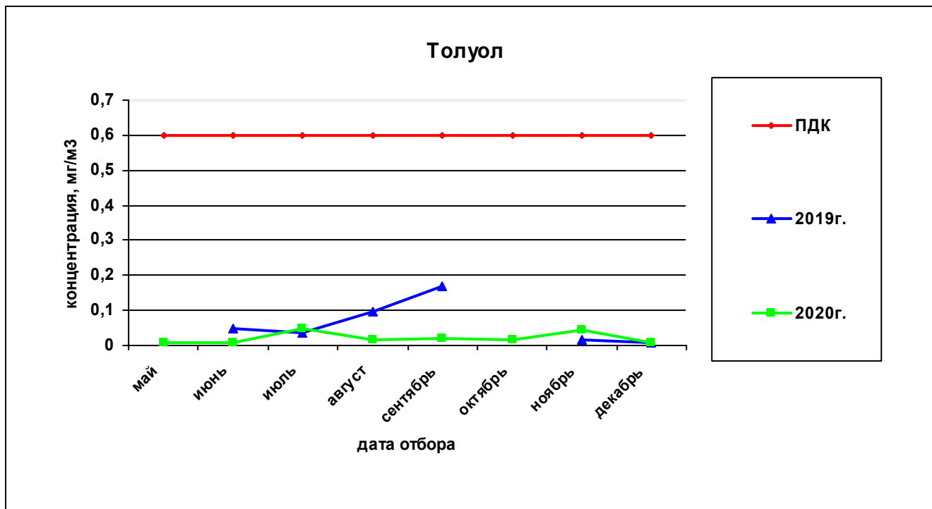
Рисунок 62— Сравнительная характеристика изменения концентрации толуола в атмосферном воздухе у домов по ул. Вавилова, 21 – Малкова, 22 за 2019 и 2020гг.
