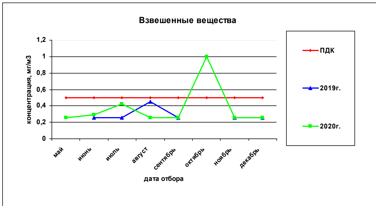
Рисунок 58— Сравнительная характеристика изменения концентрации взвешенных веществ в атмосферном воздухе у домов по ул. Вавилова, 21 – Малкова, 22 за 2019 и 2020гг.
