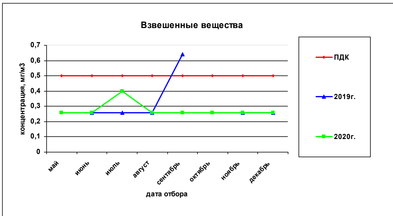
Рисунок 42— Сравнительная характеристика изменения концентрации взвешенных веществ в атмосферном воздухе на ул. Строителей, 16 за 2019 и 2020гг.
