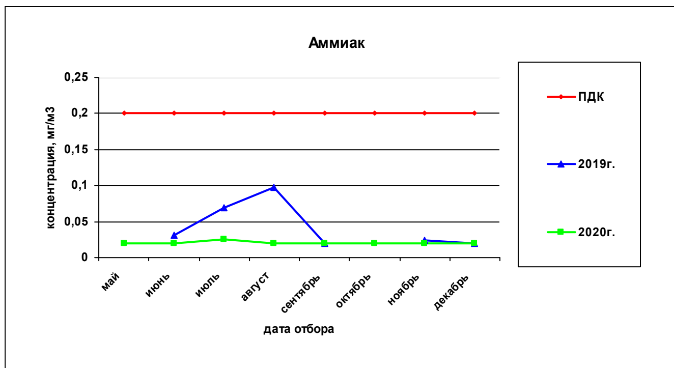
Рисунок 22— Сравнительная характеристика изменения концентрации аммиака в атмосферном воздухе на ул. Костычева за 2019 и 2020гг.
