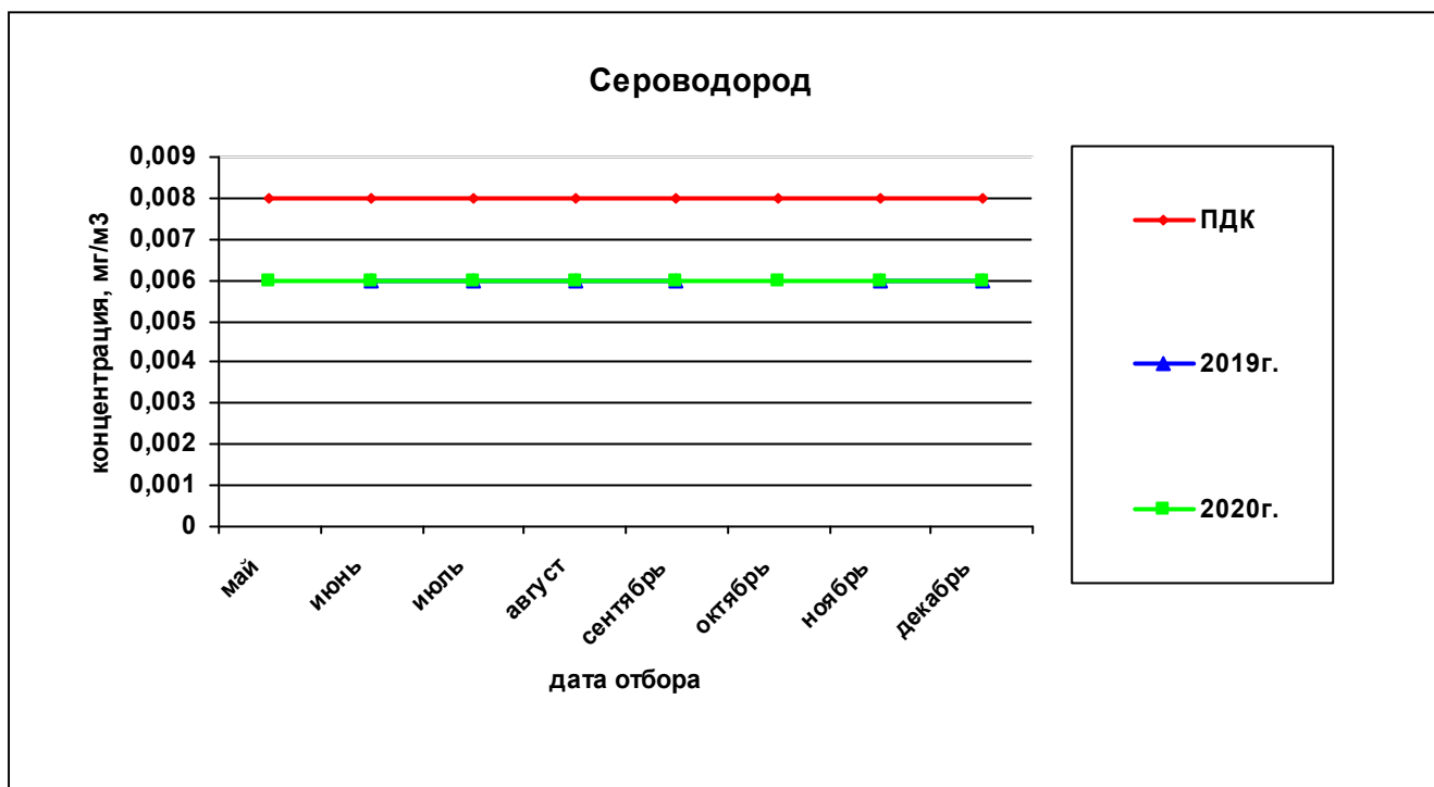
Рисунок 53— Сравнительная характеристика изменения концентрации сероводорода в атмосферном воздухе у домов по ул. Вавилова, 21 – Малкова, 22 за 2019 и 2020гг.
