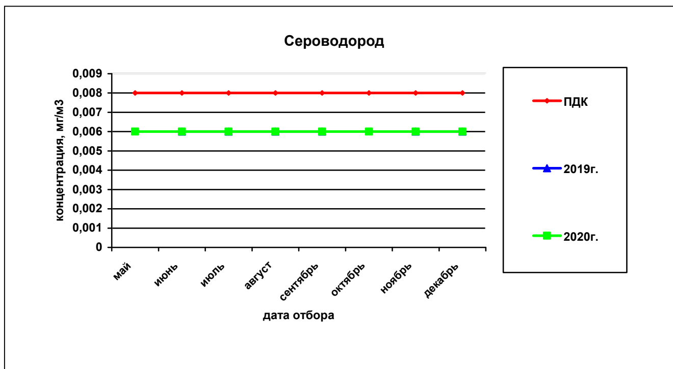
Рисунок 69— Сравнительная характеристика изменения концентрации сероводорода в атмосферном воздухе на ул.Петропавловская,185 за 2019 и 2020гг.
