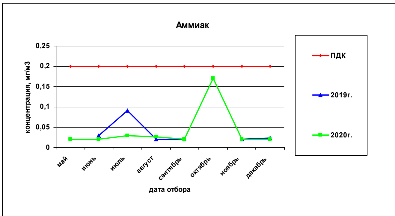
Рисунок 54— Сравнительная характеристика изменения концентрации аммиака в атмосферном воздухе у домов по ул. Вавилова, 21 – Малкова, 22 за 2019 и 2020гг.
