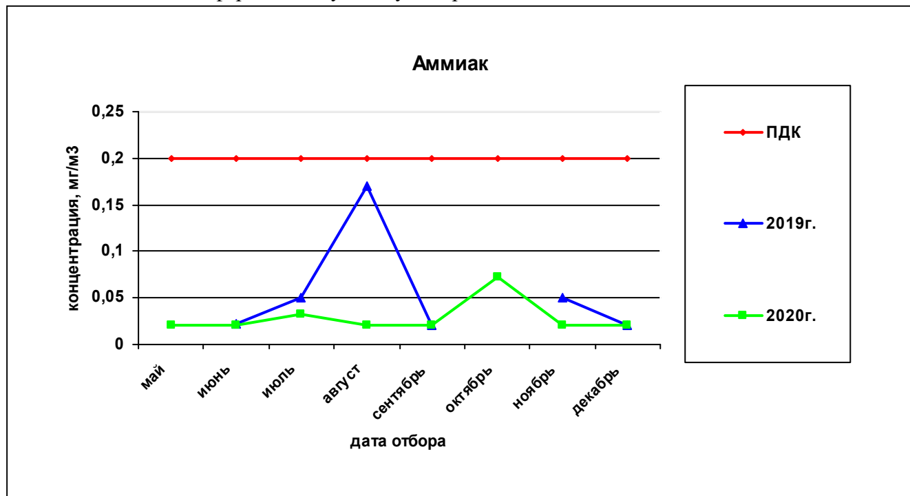
Рисунок 38— Сравнительная характеристика изменения концентрации аммиака в атмосферном воздухе на ул. Строителей, 16 за 2019 и 2020гг.
