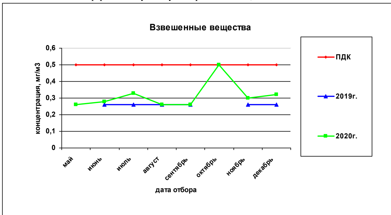
Рисунок 74— Сравнительная характеристика изменения концентрации взвешенных веществ в атмосферном воздухе на ул.Петропавловская,185 за 2019 и 2020гг.
