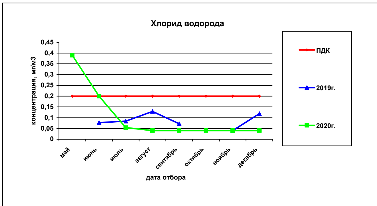
Рисунок 35— Сравнительная характеристика изменения концентрации хлорида водорода в атмосферном воздухе на ул. Строителей, 16 за 2019 и 2020гг.
