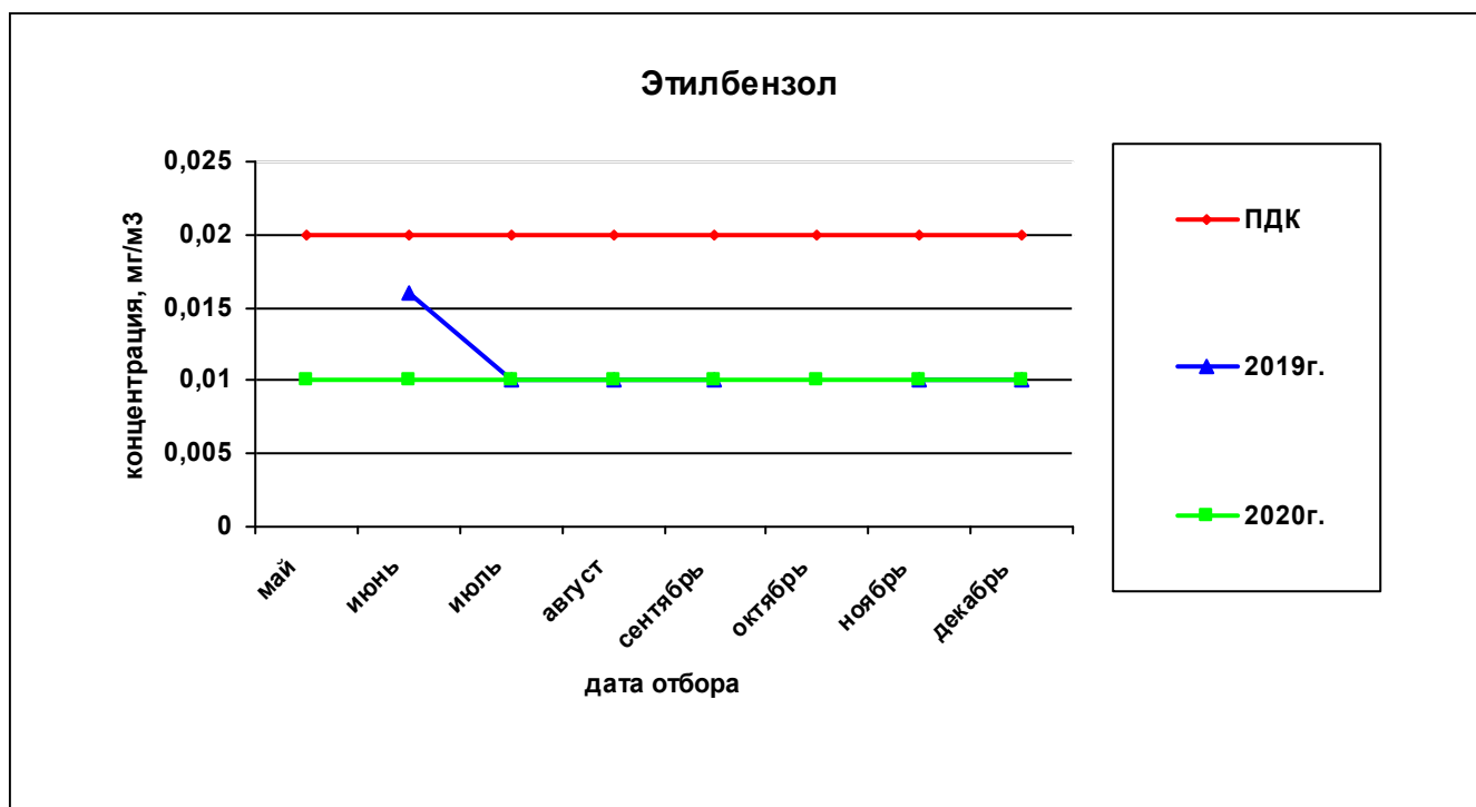
Рисунок 64— Сравнительная характеристика изменения концентрации ЭТИЛБЕНЗОЛА в атмосферном воздухе домов по ул. Вавилова, 21 – Малкова, 22 за 2019 и 2020гг.
