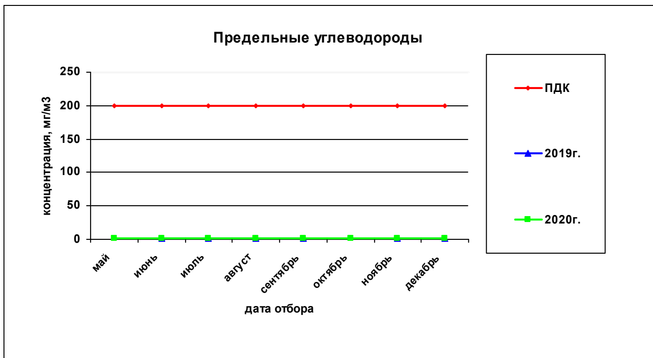
Рисунок 44— Сравнительная характеристика изменения концентрации предельных углеводородов в атмосферном воздухе на ул. Строителей, 16 за 2019 и 2020гг.
