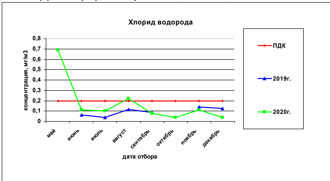
Рисунок 51— Сравнительная характеристика изменения концентрации хлорида водорода в атмосферном воздухе у домов по ул. Вавилова, 21 – Малкова, 22 за 2019 и 2020гг.
