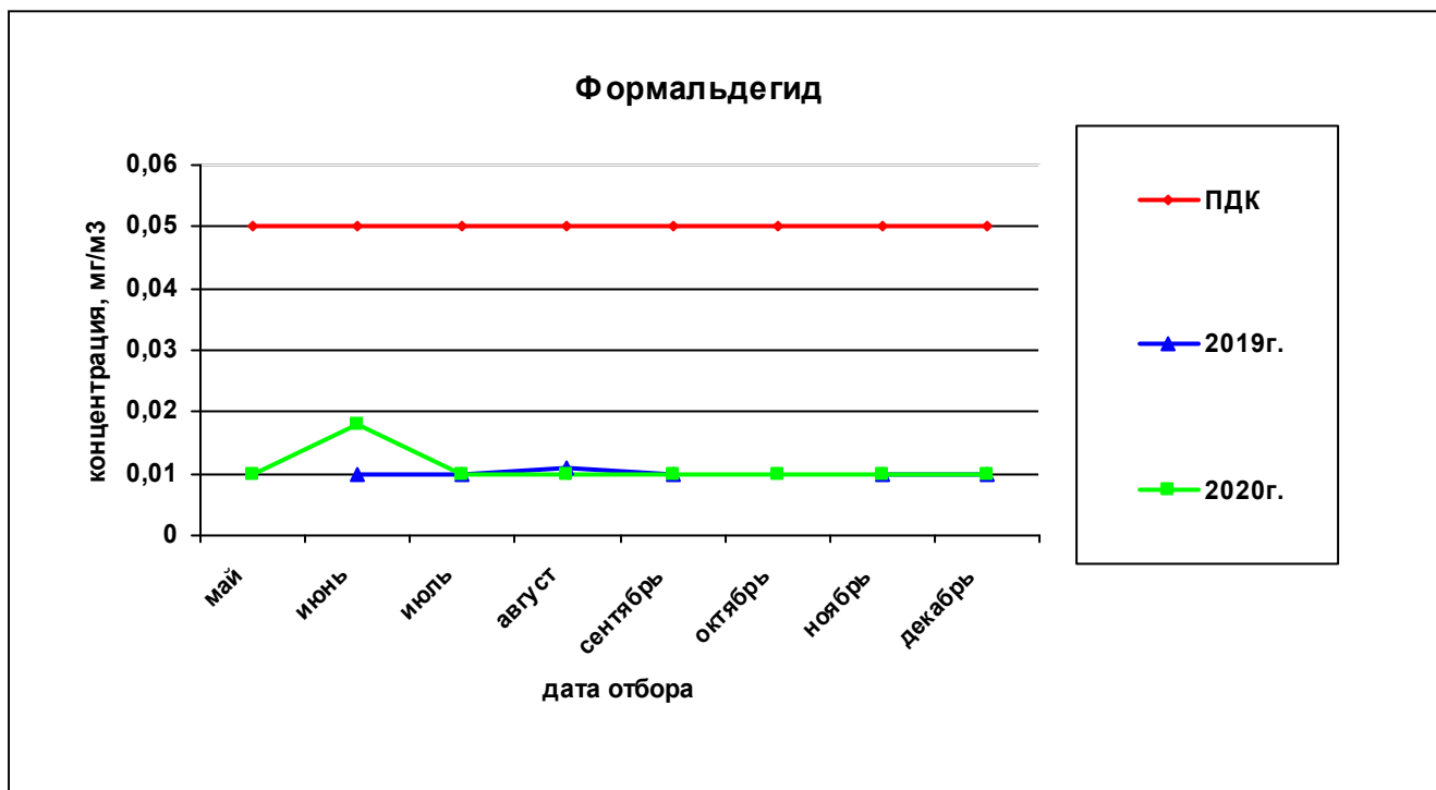
Рисунок 41— Сравнительная характеристика изменения концентрации формальдегида в атмосферном воздухе на ул. Строителей, 16 за 2019 и 2020гг.
