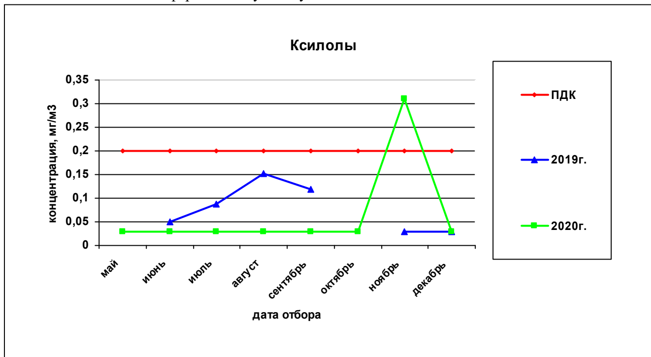
Рисунок 31— Сравнительная характеристика изменения концентрации КСИЛОЛОВ в атмосферном воздухе на ул. Костычева за 2019 и 2020гг.
