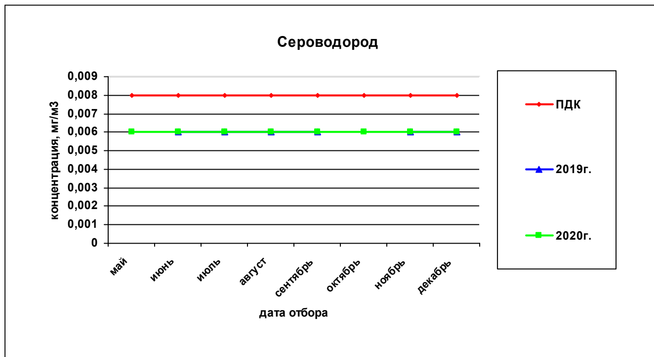
Рисунок 21— Сравнительная характеристика изменения концентрации сероводорода в атмосферном воздухе на ул. Костычева за 2019 и 2020гг.
