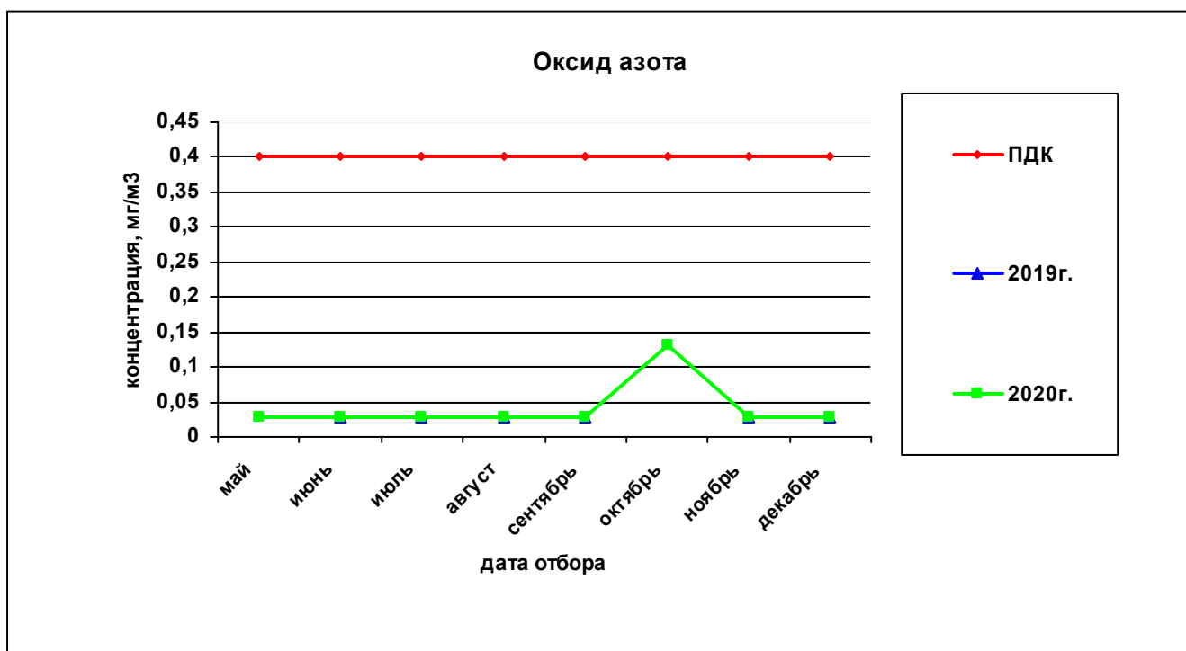
Рисунок 50— Сравнительная характеристика изменения концентрации оксида азота в атмосферном воздухе у домов по ул. Вавилова, 21 – Малкова, 22 за 2019 и 2020гг.
