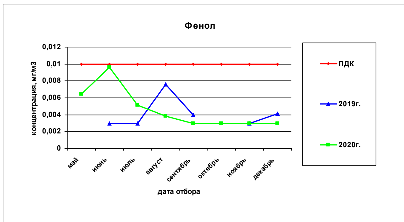
Рисунок 40— Сравнительная характеристика изменения концентрации фенола в атмосферном воздухе на ул. Строителей, 16 за 2019 и 2020гг.
