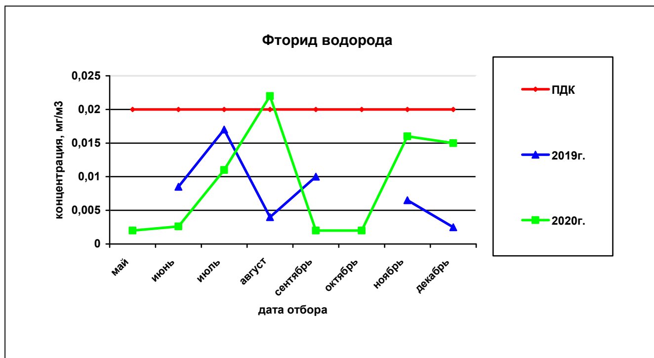
Рисунок 75— Сравнительная характеристика изменения концентрации фторида водорода в атмосферном воздухе на ул.Петропавловская,185 за 2019 и 2020гг.
