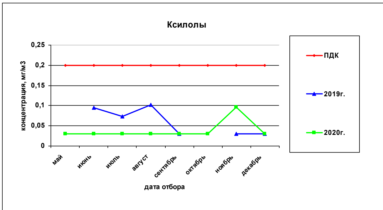
Рисунок 47— Сравнительная характеристика изменения концентрации КСИЛОЛОВ в атмосферном воздухе на ул. Строителей, 16 за 2019 и 2020гг.
