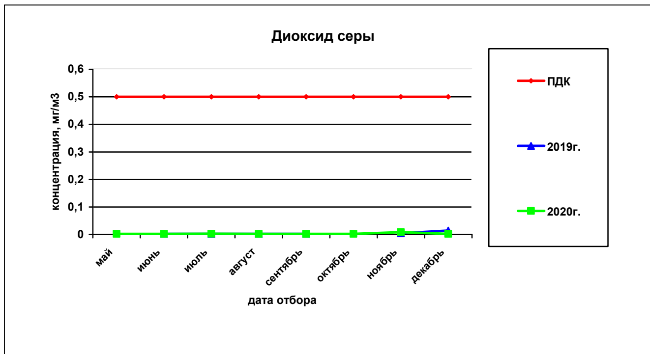
Рисунок 36— Сравнительная характеристика изменения концентрации диоксида серы в атмосферном воздухе на ул. Строителей, 16 за 2019 и 2020гг.
