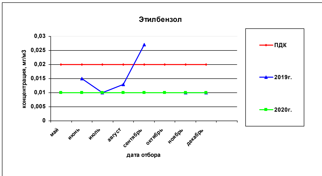
Рисунок 32— Сравнительная характеристика изменения концентрации ЭТИЛБЕНЗОЛА в атмосферном воздухе на ул. Костычева за 2019 и 2020гг.
