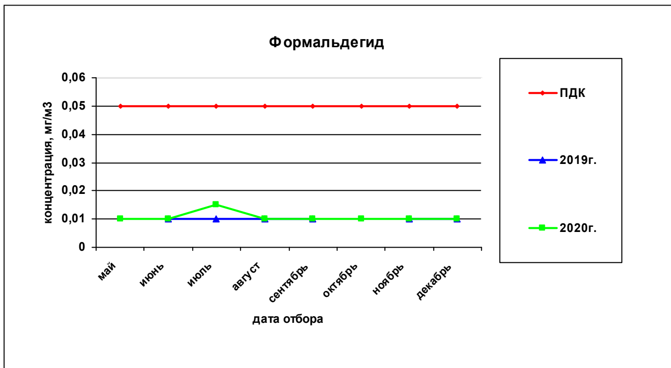
Рисунок 57— Сравнительная характеристика изменения концентрации формальдегида в атмосферном воздухе у домов по ул. Вавилова, 21 – Малкова, 22 за 2019 и 2020гг.
