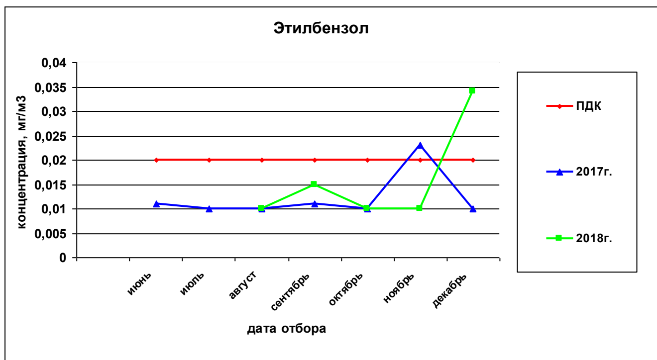
Рисунок 64— Сравнительная характеристика изменения концентрации этилбензола в атмосферном воздухе домов по ул. Вавилова, 21 – Малкова, 22 за 2017 и 2018гг.
