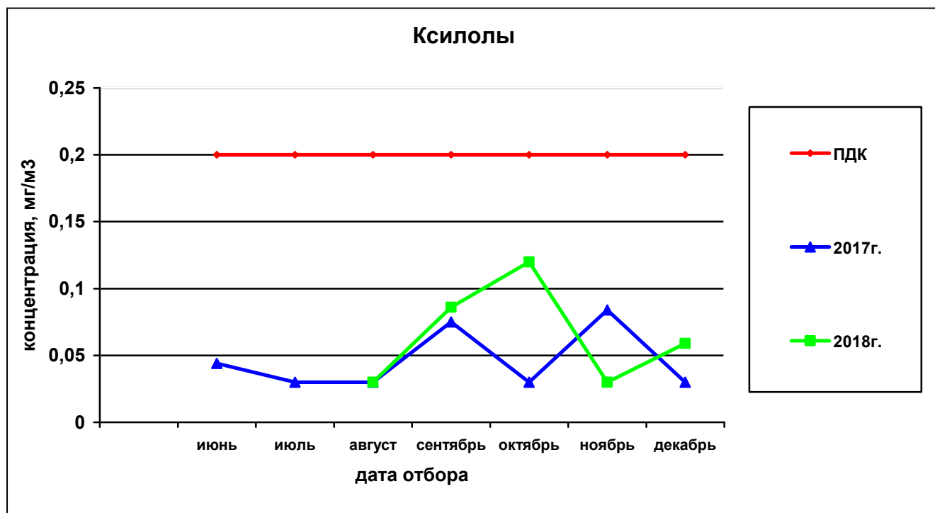
Рисунок 63— Сравнительная характеристика изменения концентрации ксилолов в атмосферном воздухе у домов по ул. Вавилова, 21 – Малкова, 22 за 2017 и 2018гг.
