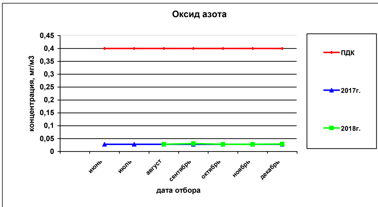
Рисунок 18— Сравнительная характеристика изменения концентрации оксида азота в атмосферном воздухе на ул. Костычева за 2017 и 2018гг.
