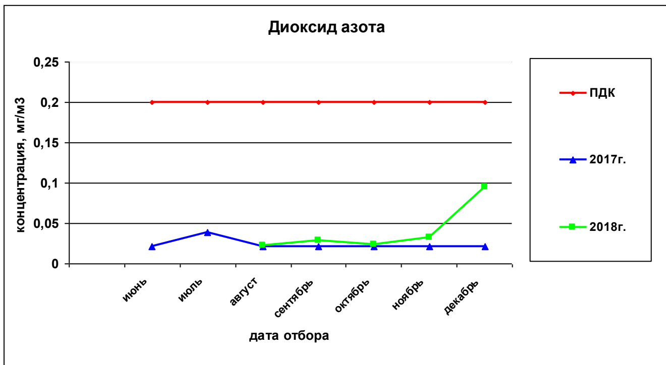
Рисунок 33— Сравнительная характеристика изменения концентрации диоксида азота в атмосферном воздухе на ул. Строителей за 2017 и 2018гг.
