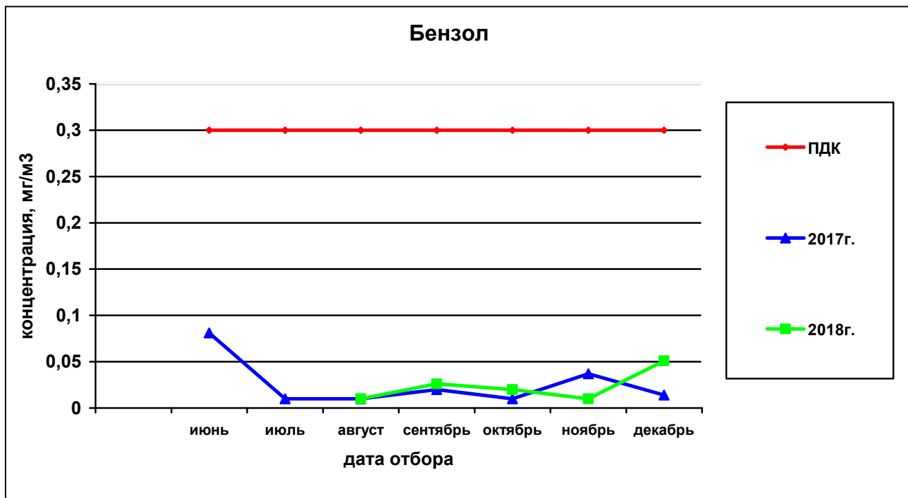
Рисунок 29— Сравнительная характеристика изменения концентрации бензола в атмосферном воздухе на ул. Костычева за 2017и 2018гг.
