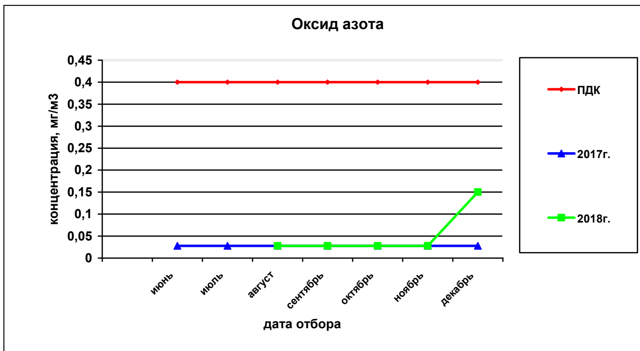
Рисунок 34— Сравнительная характеристика изменения концентрации оксида азота в атмосферном воздухе на ул. Строителей за 2017 и 2018гг.
