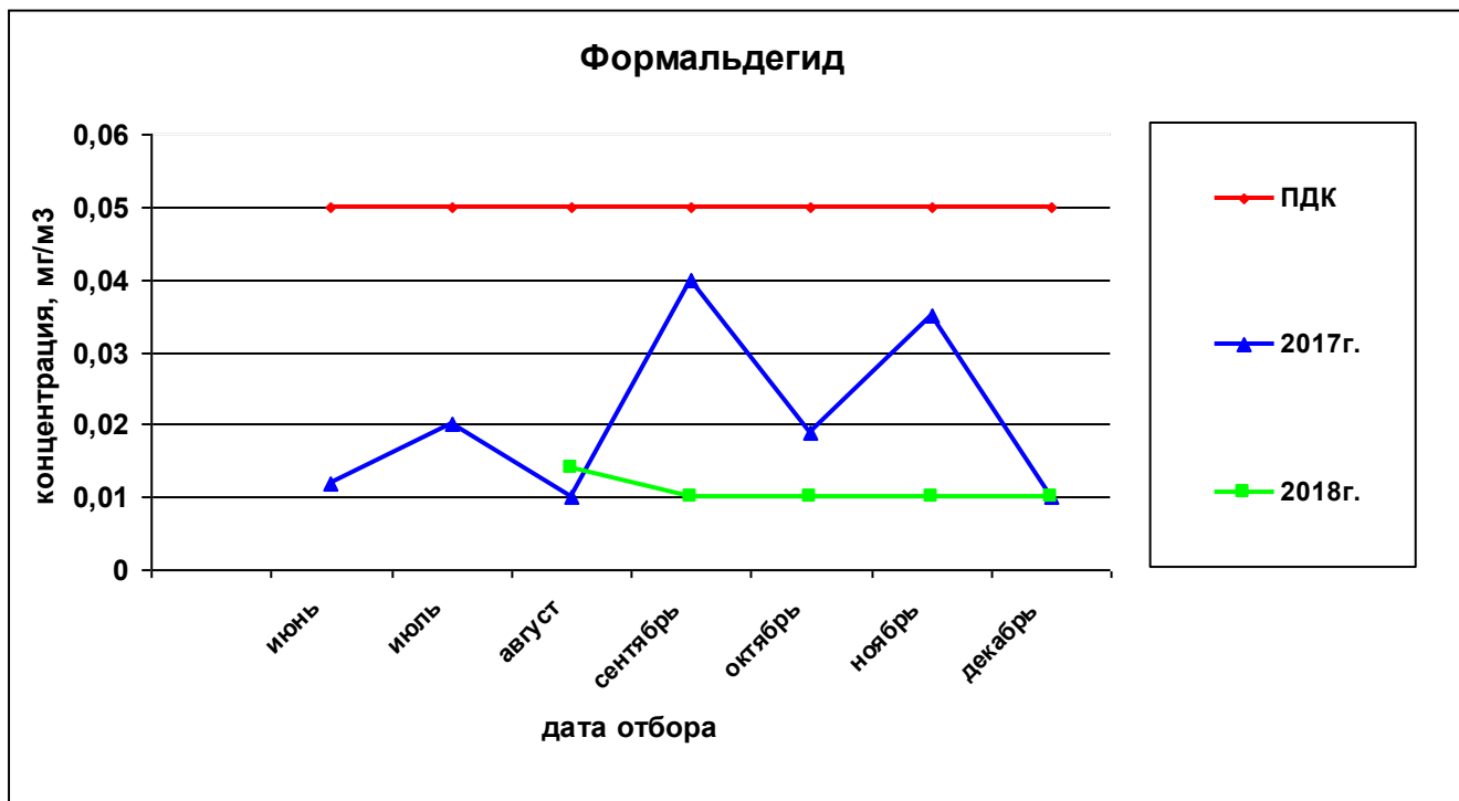
Рисунок 25— Сравнительная характеристика изменения концентрации формальдегида в атмосферном воздухе на ул. Костычева за 2017 и 2018гг.
