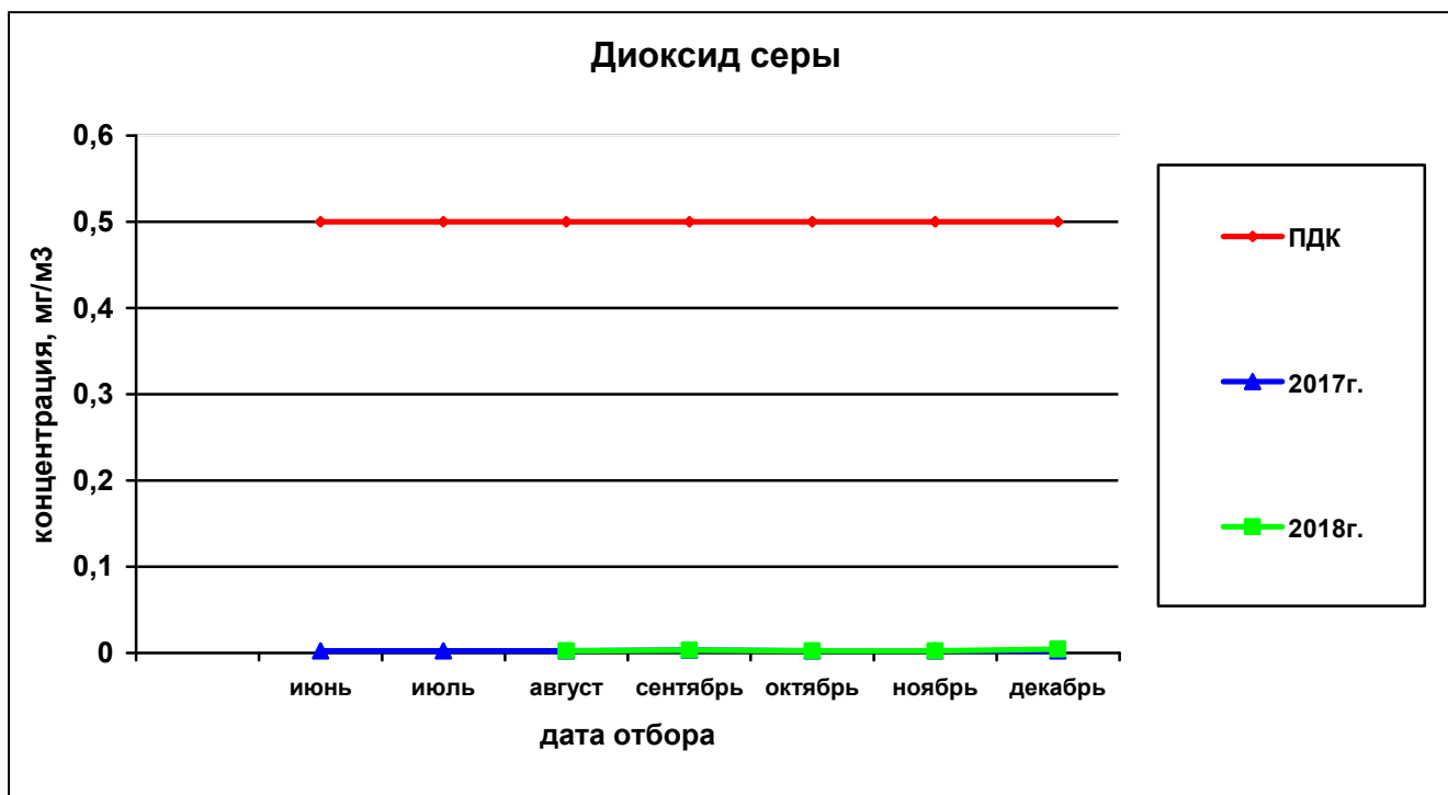
Рисунок 20— Сравнительная характеристика изменения концентрации диоксида серы в атмосферном воздухе на ул. Костычева за 2017 и 2018гг.
