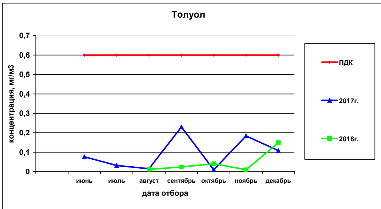
Рисунок 30— Сравнительная характеристика изменения концентрации толуола в атмосферном воздухе на ул. Костычева за 2017 и 2018гг.
