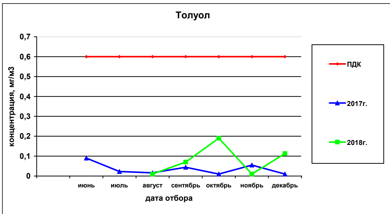
Рисунок 78— Сравнительная характеристика изменения концентрации толуола в атмосферном воздухе на ул.Петропавловская,185 за 2017 и 2018гг.
