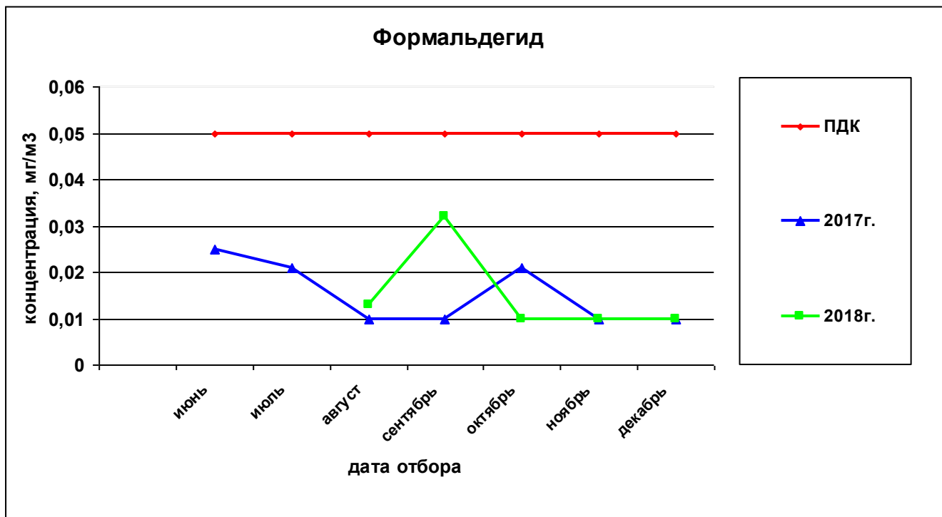
Рисунок 41— Сравнительная характеристика изменения концентрации формальдегида в атмосферном воздухе на ул. Строителей за 2017 и 2018гг.
