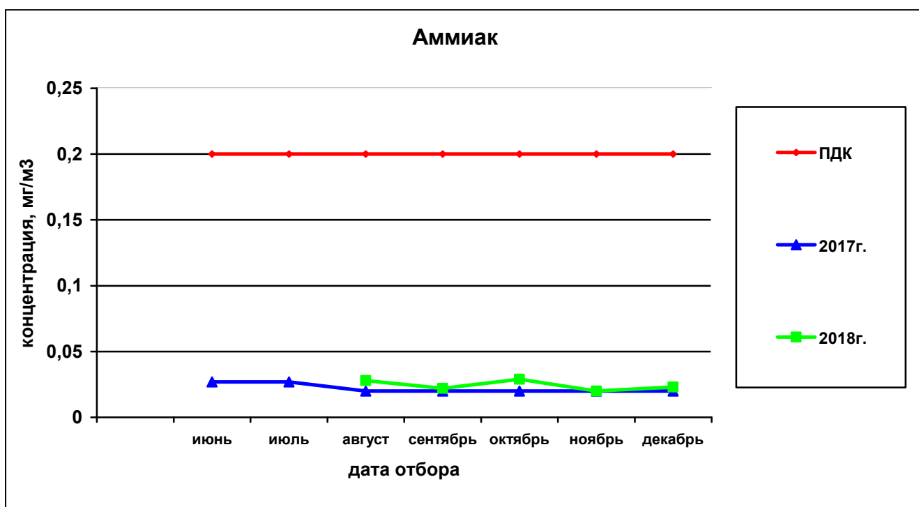
Рисунок 22— Сравнительная характеристика изменения концентрации аммиака в атмосферном воздухе на ул. Костычева за 2017 и 2018гг.
