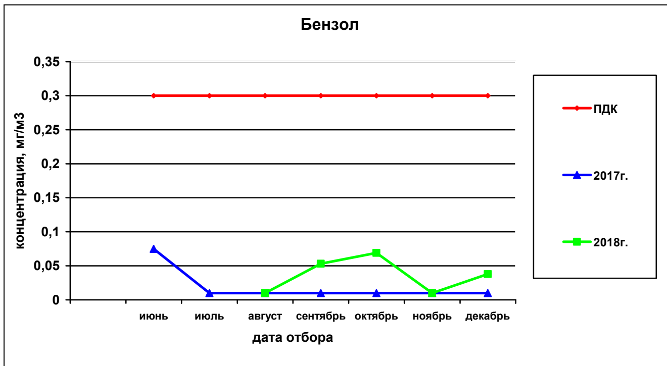
Рисунок 77— Сравнительная характеристика изменения концентрации бензола в атмосферном воздухе на ул.Петропавловская,185 за 2017 и 2018гг.
