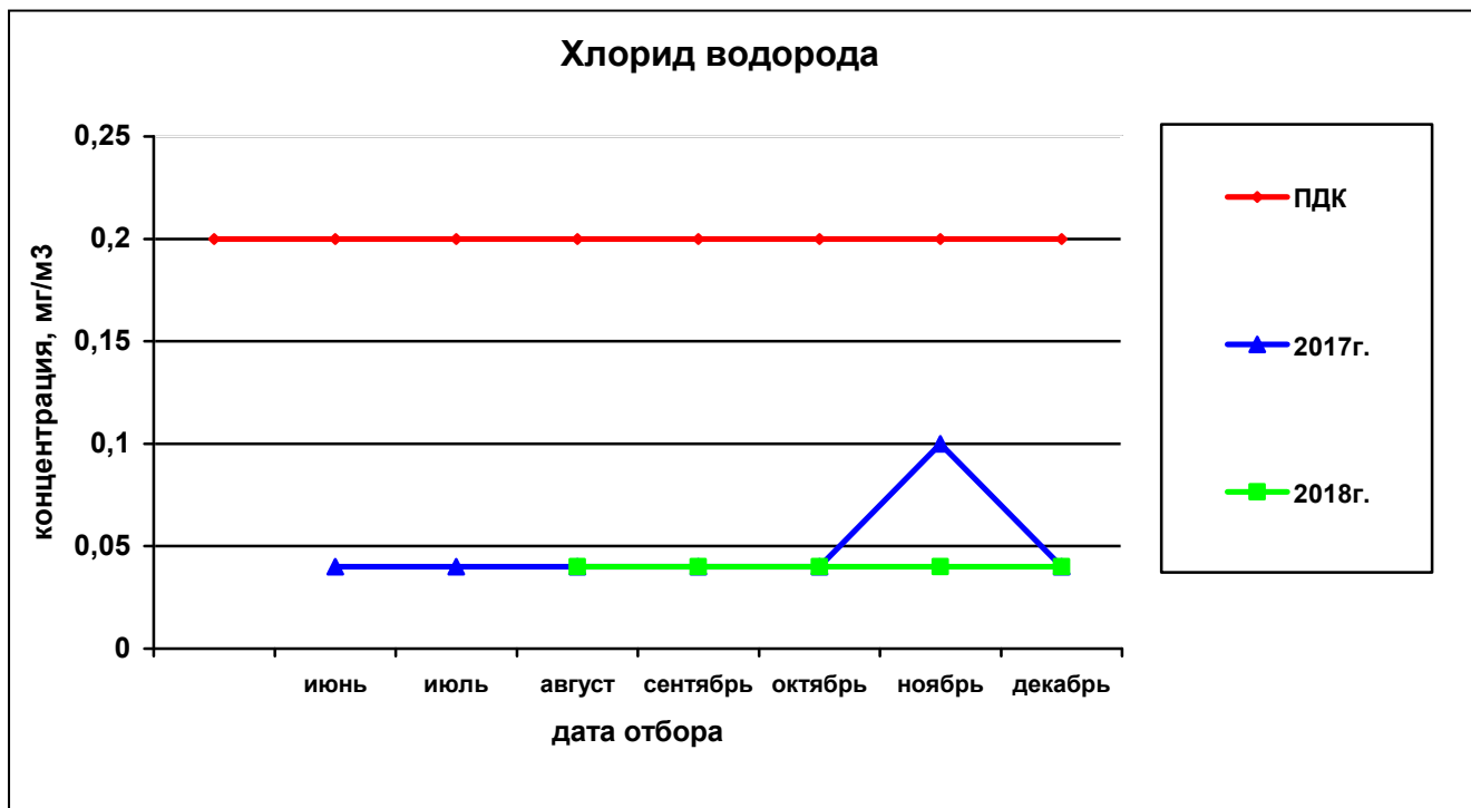
Рисунок 35— Сравнительная характеристика изменения концентрации хлорида водорода в атмосферном воздухе на ул. Строителей за 2017 и 2018гг.
