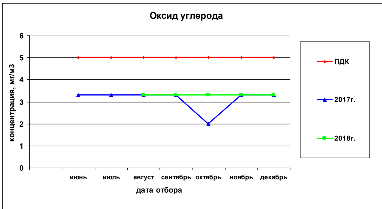
Рисунок 39— Сравнительная характеристика изменения концентрации оксида углерода в атмосферном воздухе на ул. Строителей за 2017 и 2018гг.
