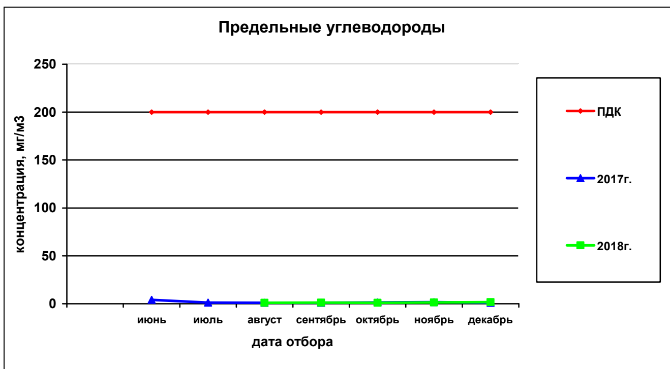
Рисунок 44— Сравнительная характеристика изменения концентрации предельных углеводородов в атмосферном воздухе на ул. Строителей за 2017 и 2018гг.
