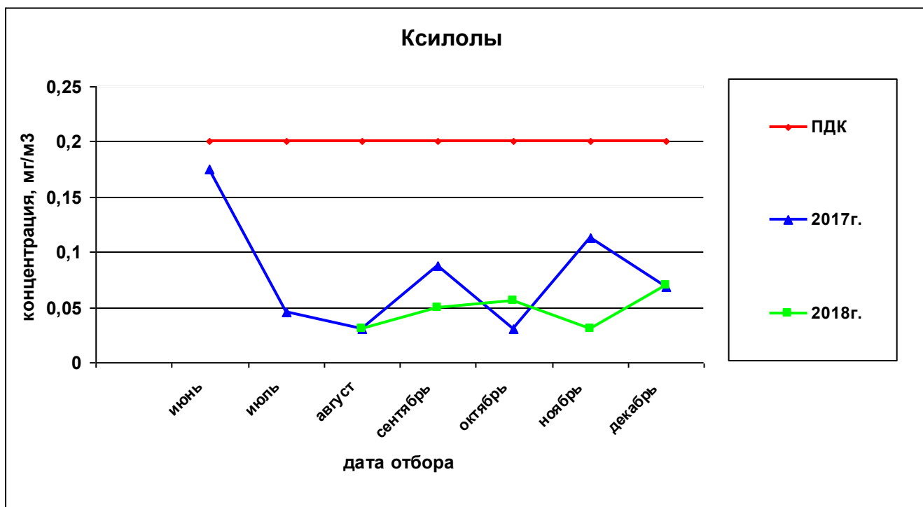
Рисунок 31— Сравнительная характеристика изменения концентрации ксилолов в атмосферном воздухе на ул. Костычева за 2017 и 2018гг.
