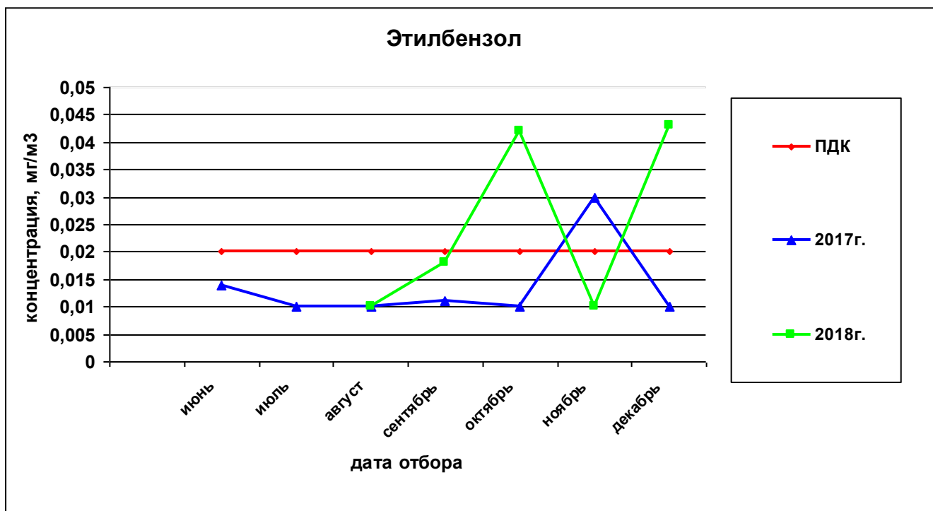
Рисунок 48— Сравнительная характеристика изменения концентрации этилбензола в атмосферном воздухе на ул. Строителей за 2017 и 2018гг.
