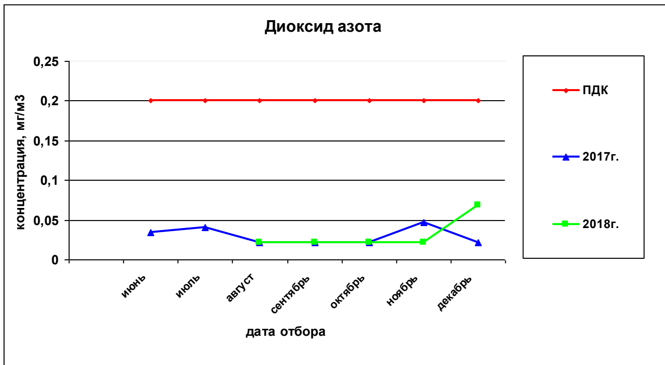
Рисунок 17— Сравнительная характеристика изменения концентрации диоксида азота в атмосферном воздухе на ул. Костычева за 2017 и 2018гг.
