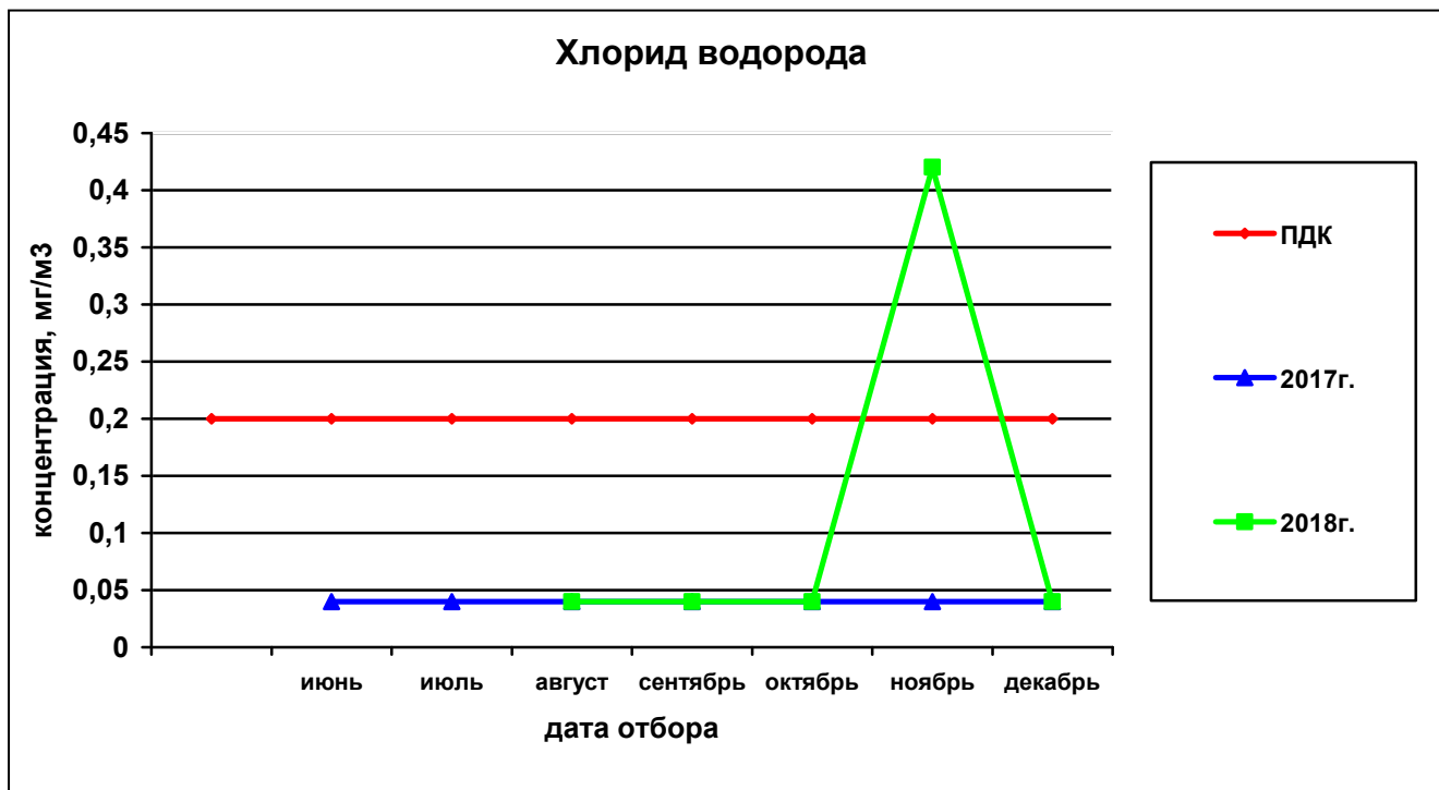
Рисунок 19— Сравнительная характеристика изменения концентрации хлорида водорода в атмосферном воздухе на ул. Костычева за 2017 и 2018гг.
