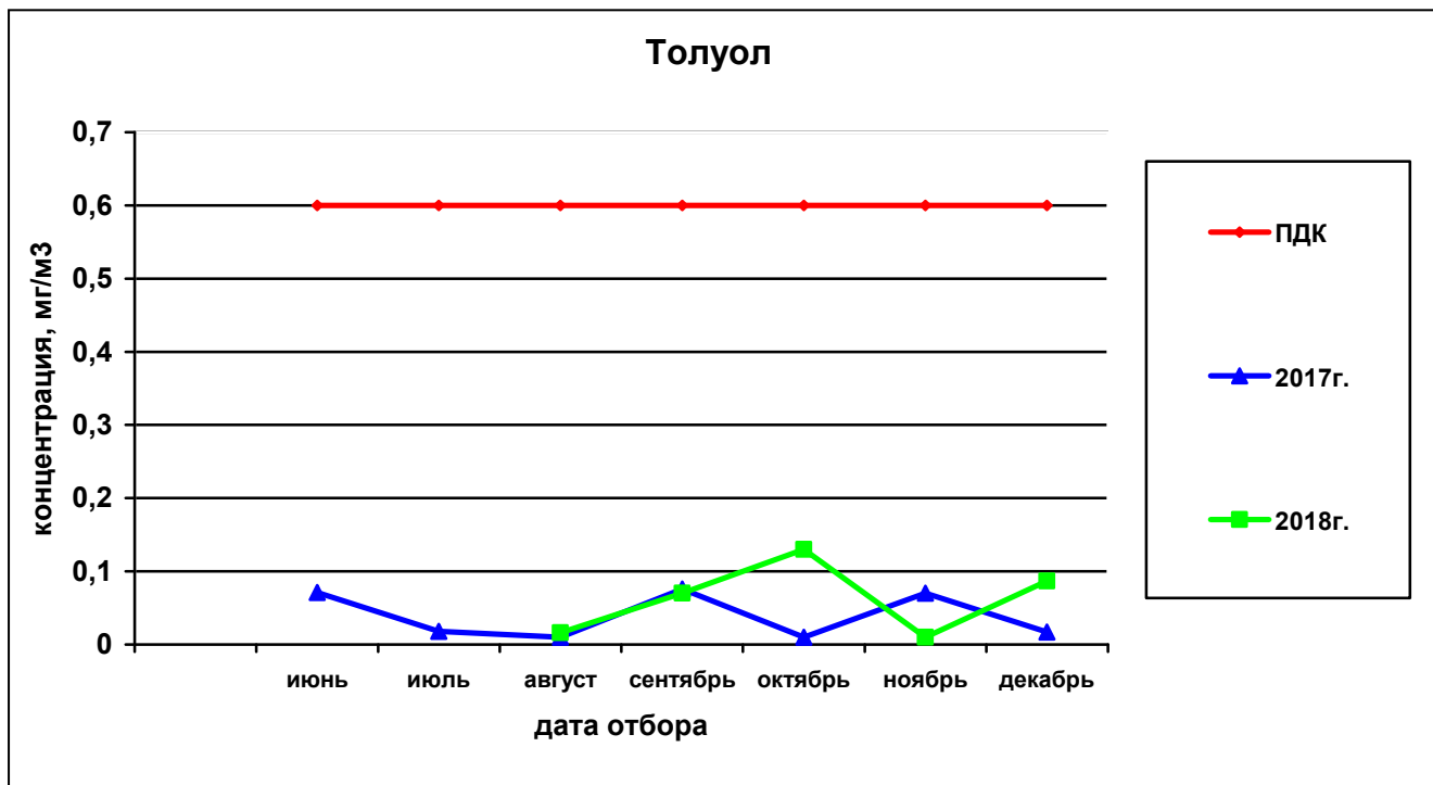
Рисунок 62— Сравнительная характеристика изменения концентрации толуола в атмосферном воздухе у домов по ул. Вавилова, 21 – Малкова, 22 за 2017 и 2018гг.
