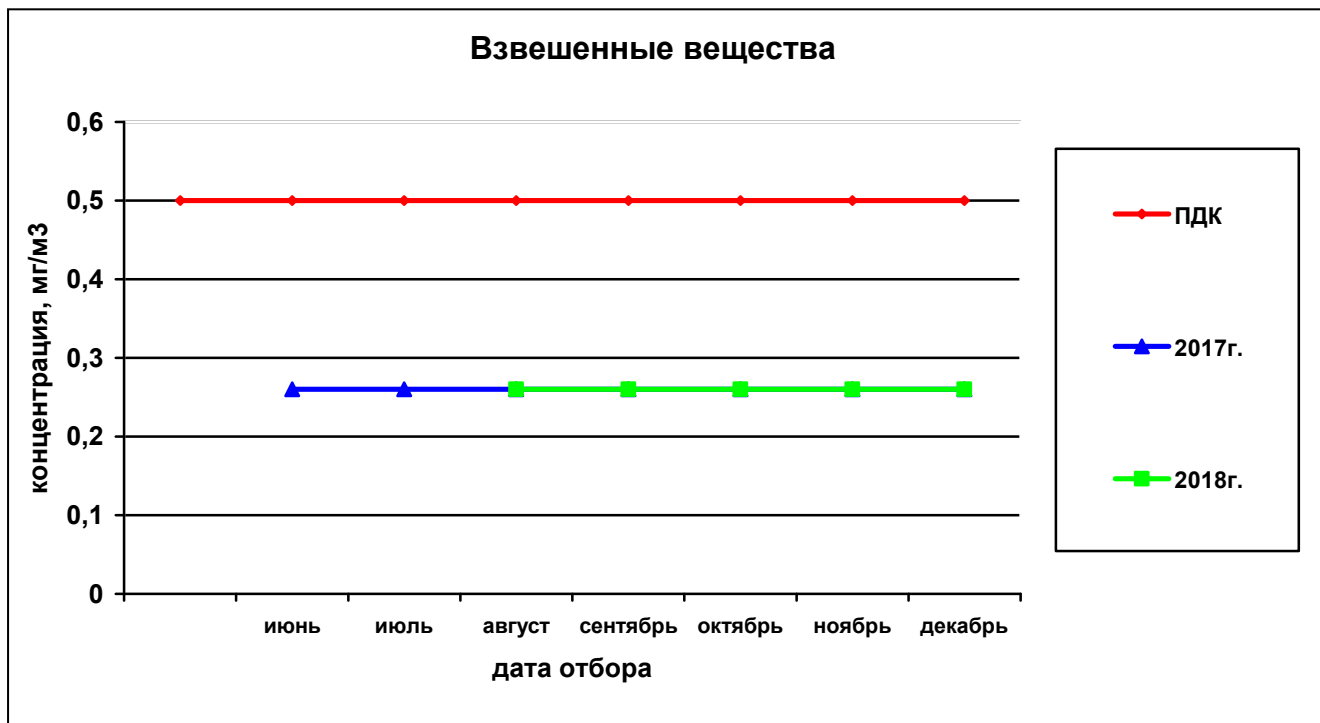
Рисунок 42— Сравнительная характеристика изменения концентрации взвешенных веществ в атмосферном воздухе на ул. Строителей за 2017 и 2018гг.
