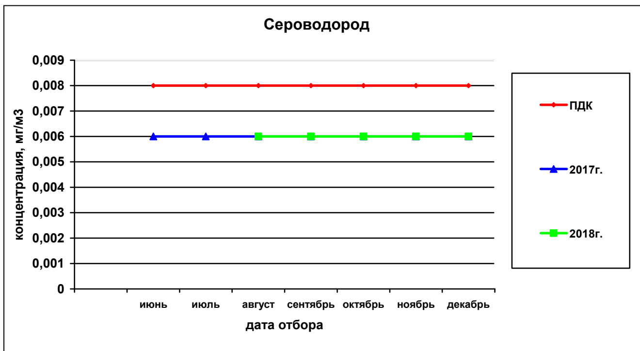
Рисунок 53— Сравнительная характеристика изменения концентрации сероводорода в атмосферном воздухе у домов по ул. Вавилова, 21 – Малкова, 22 за 2017 и 2018гг.
