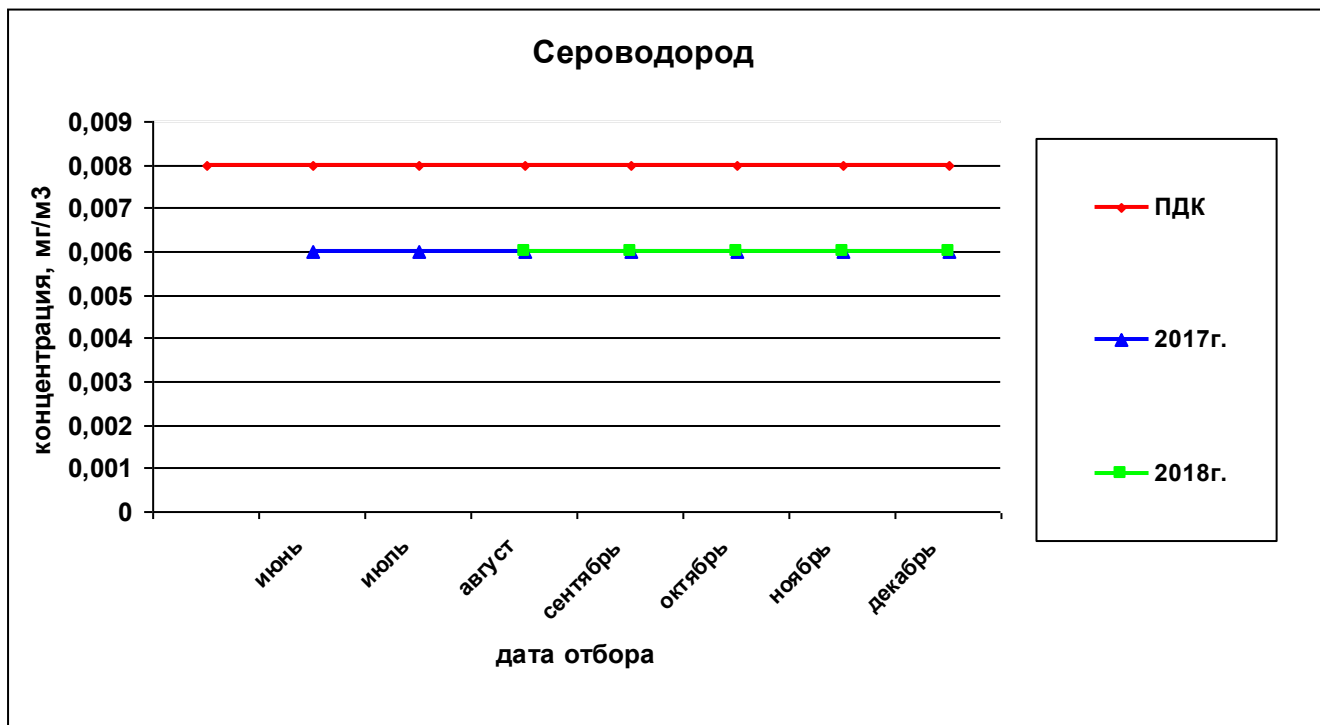
Рисунок 37— Сравнительная характеристика изменения концентрации сероводорода в атмосферном воздухе на ул. Строителей за 2017 и 2018гг.
