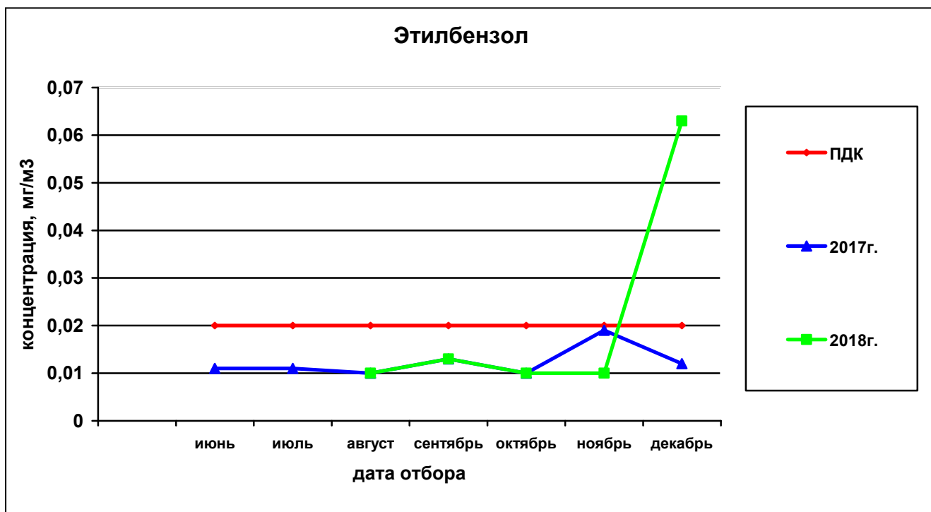
Рисунок 32— Сравнительная характеристика изменения концентрации этилбензола в атмосферном воздухе на ул. Костычева за 2017 и 2018гг.
