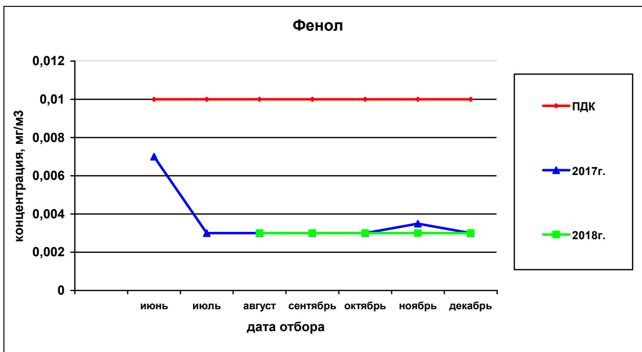
Рисунок 72— Сравнительная характеристика изменения концентрации фенола в атмосферном воздухе на ул.Петропавловская,185 за 2017 и 2018гг.
