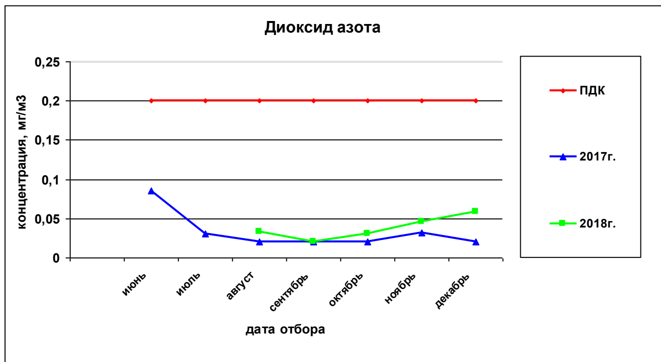
Рисунок 65— Сравнительная характеристика изменения концентрации диоксида азота в атмосферном воздухе на ул.Петропавловская,185 за 2017 и 2018гг.
