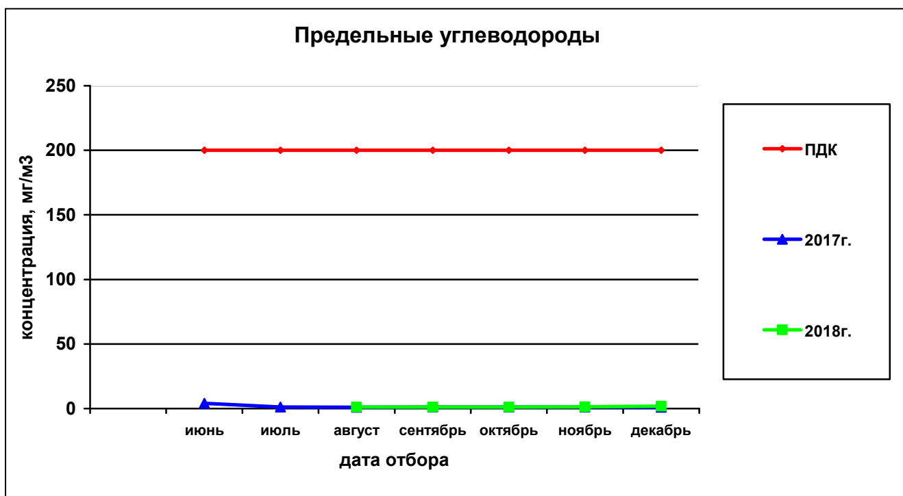
Рисунок 60— Сравнительная характеристика изменения концентрации предельных углеводородов в атмосферном воздухе у домов по ул. Вавилова, 21 – Малкова, 22 за 2017 и 2018гг.
