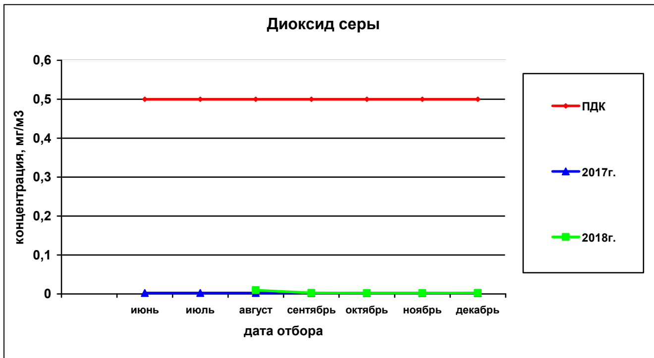
Рисунок 52— Сравнительная характеристика изменения концентрации диоксида серы в атмосферном воздухе у домов по ул. Вавилова, 21 – Малкова, 22 за 2017 и 2018гг.
