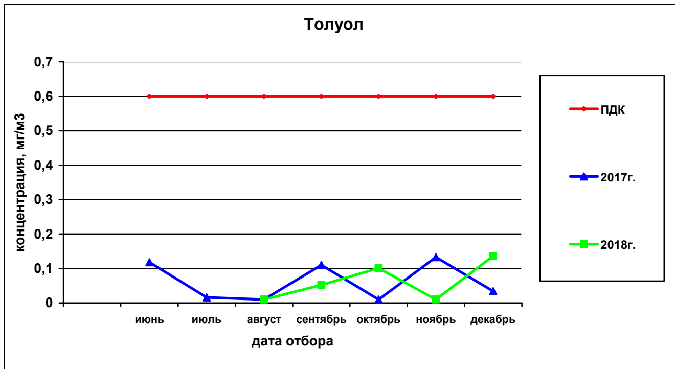
Рисунок 46— Сравнительная характеристика изменения концентрации толуола в атмосферном воздухе на ул. Строителей за 2017 и 2018гг.
