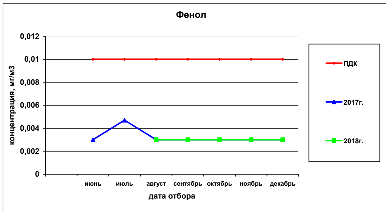
Рисунок 24— Сравнительная характеристика изменения концентрации фенола в атмосферном воздухе на ул. Костычева за 2017 и 2018гг.
