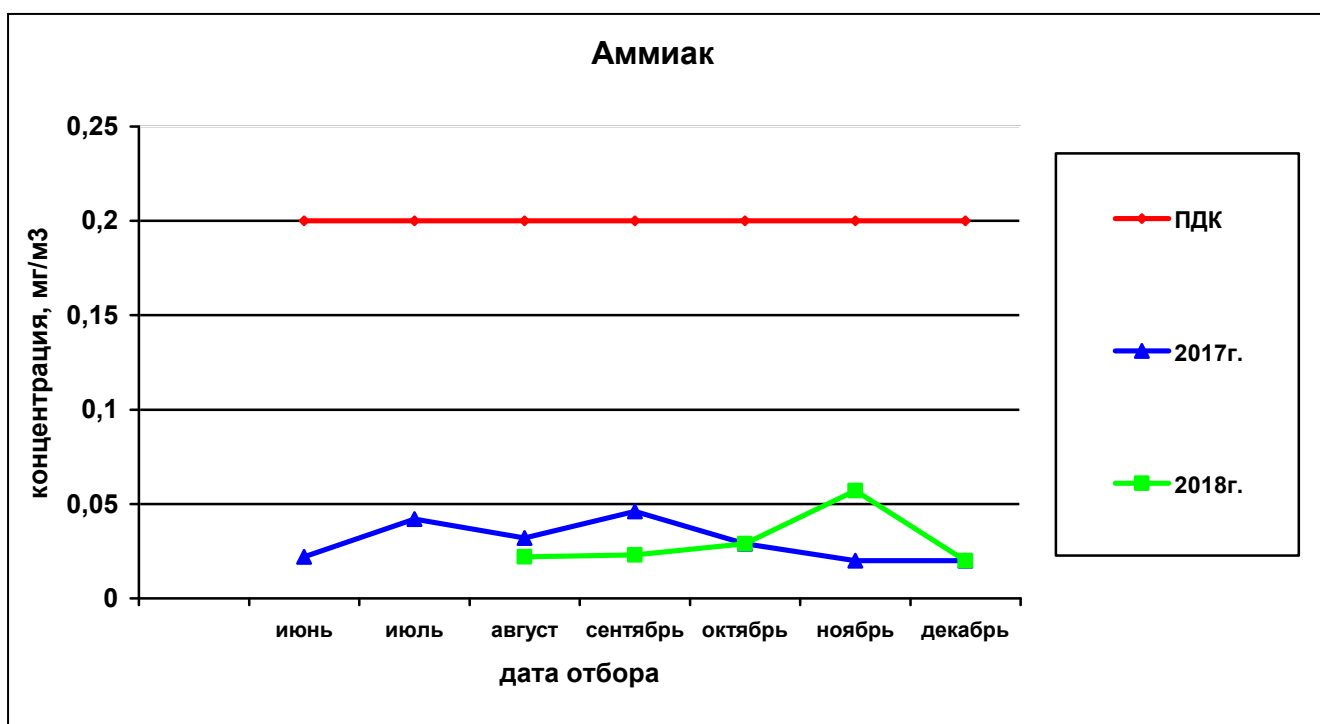
Рисунок 54— Сравнительная характеристика изменения концентрации аммиака в атмосферном воздухе у домов по ул. Вавилова, 21 – Малкова, 22 за 2017 и 2018гг.
