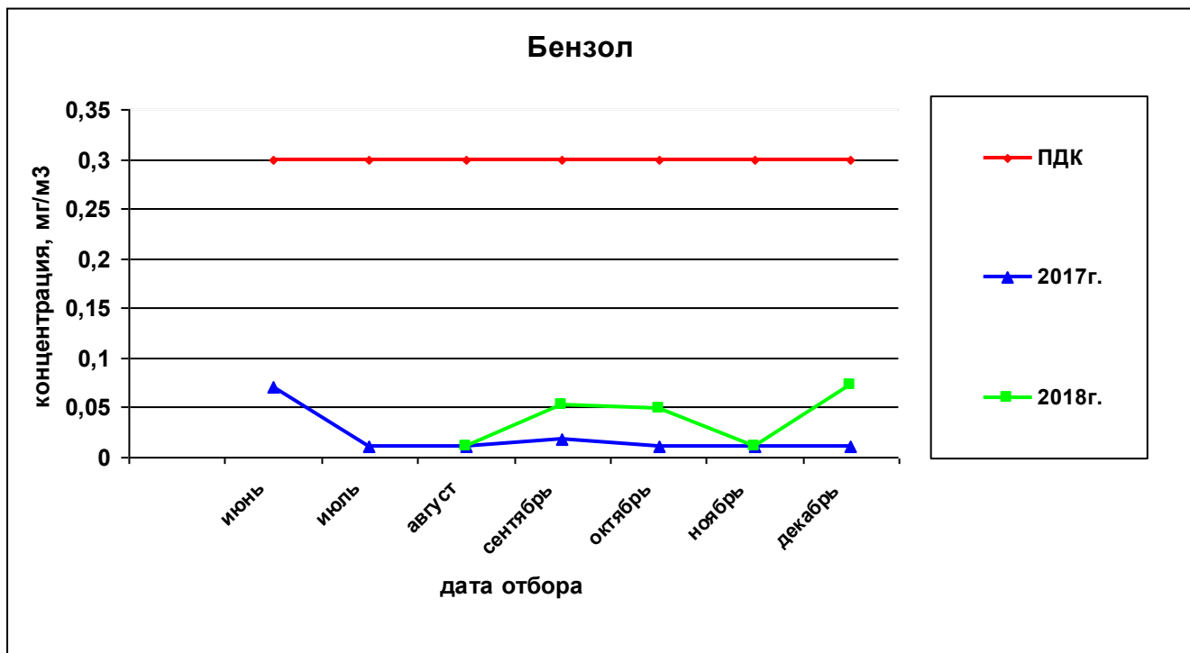
Рисунок 61— Сравнительная характеристика изменения концентрации бензола в атмосферном воздухе у домов по ул. Вавилова, 21 – Малкова, 22 за 2017 и 2018гг.
