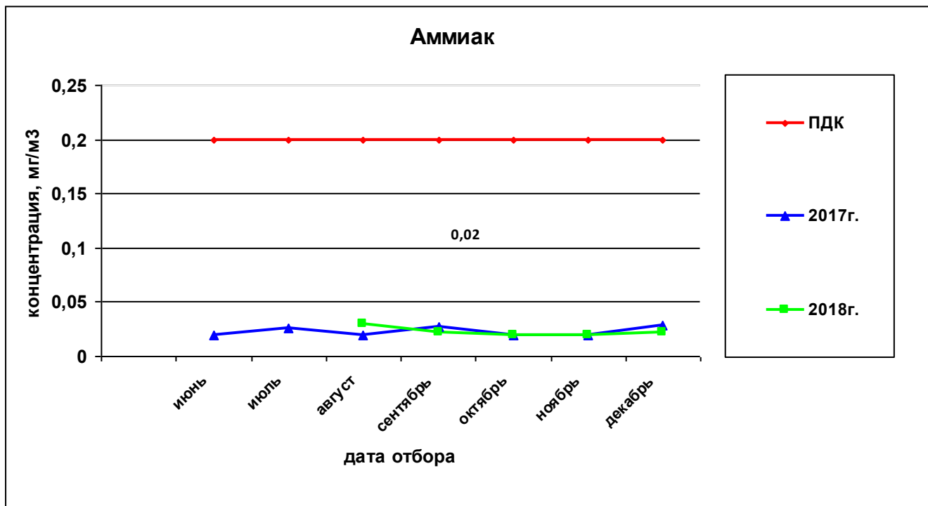
Рисунок 38— Сравнительная характеристика изменения концентрации аммиака в атмосферном воздухе на ул. Строителей за 2017 и 2018гг.
