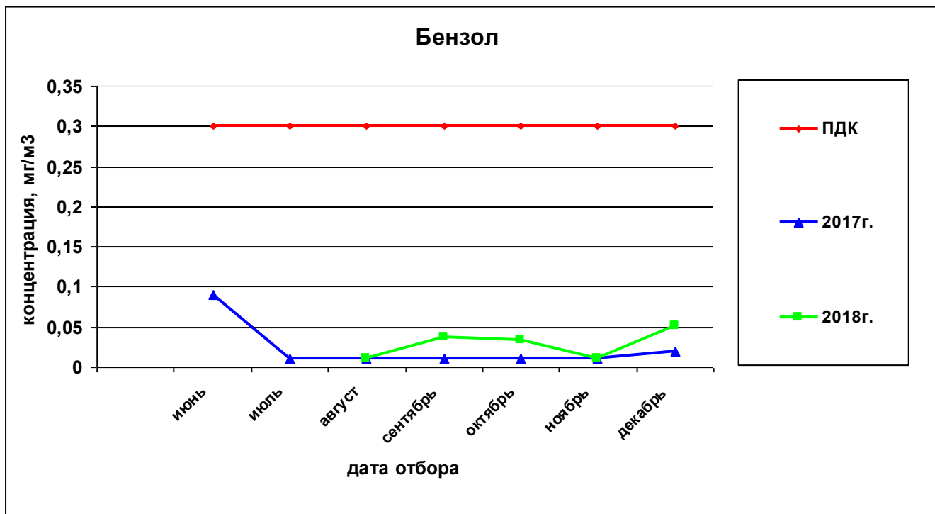
Рисунок 45— Сравнительная характеристика изменения концентрации бензола в атмосферном воздухе на ул. Строителей за 2017 и 2018гг.
