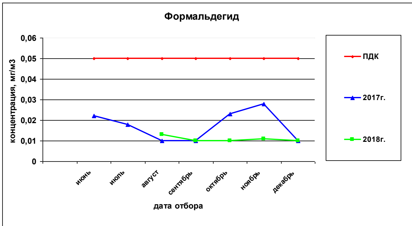
Рисунок 73— Сравнительная характеристика изменения концентрации формальдегида в атмосферном воздухе на ул.Петропавловская,185 за 2017 и 2018гг.
