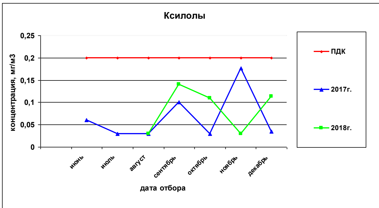
Рисунок 47— Сравнительная характеристика изменения концентрации ксилолов в атмосферном воздухе на ул. Строителей за 2017 и 2018гг.
