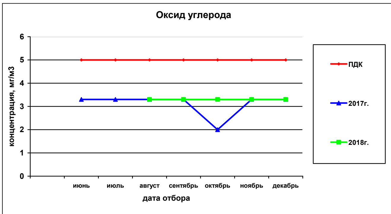
Рисунок 71— Сравнительная характеристика изменения концентрации оксида углерода в атмосферном воздухе на ул.Петропавловская,185 за 2017 и 2018гг.
