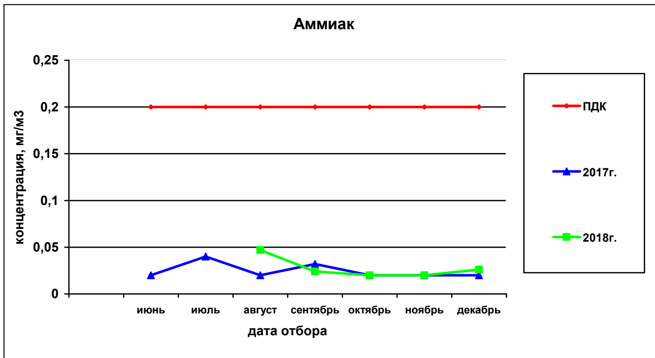
Рисунок 70— Сравнительная характеристика изменения концентрации аммиака в атмосферном воздухе на ул.Петропавловская,185 за 2017 и 2018гг.
