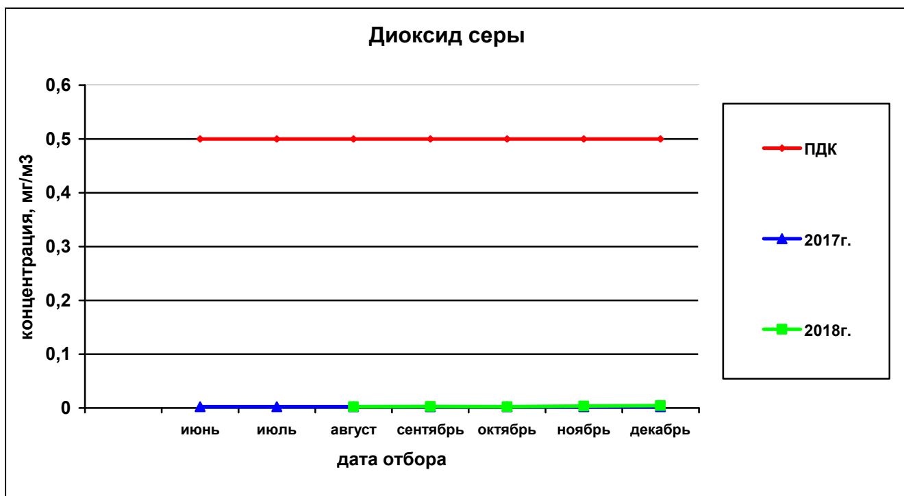
Рисунок 68— Сравнительная характеристика изменения концентрации диоксида серы в атмосферном воздухе на ул.Петропавловская,185 за 2017 и 2018гг.
