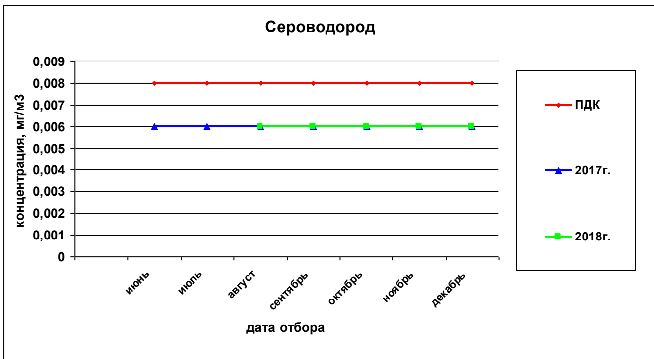
Рисунок 21— Сравнительная характеристика изменения концентрации сероводорода в атмосферном воздухе на ул. Костычева за 2017 и 2018гг.
