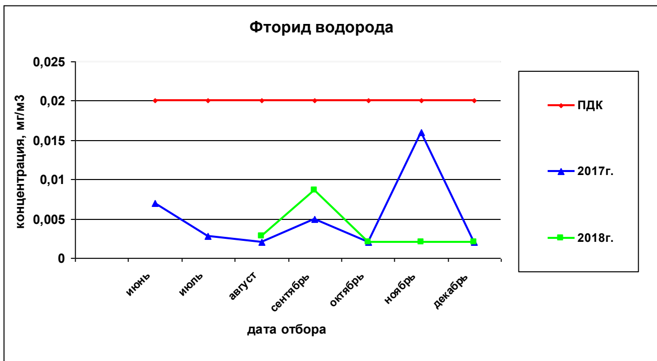
Рисунок 43— Сравнительная характеристика изменения концентрации фторида водорода в атмосферном воздухе на ул. Строителей за 2017 и 2018гг.
