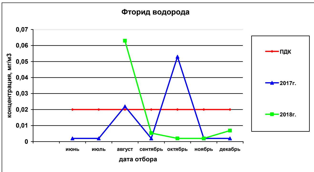
Рисунок 75— Сравнительная характеристика изменения концентрации фторида водорода в атмосферном воздухе на ул.Петропавловская,185 за 2017 и 2018гг.
