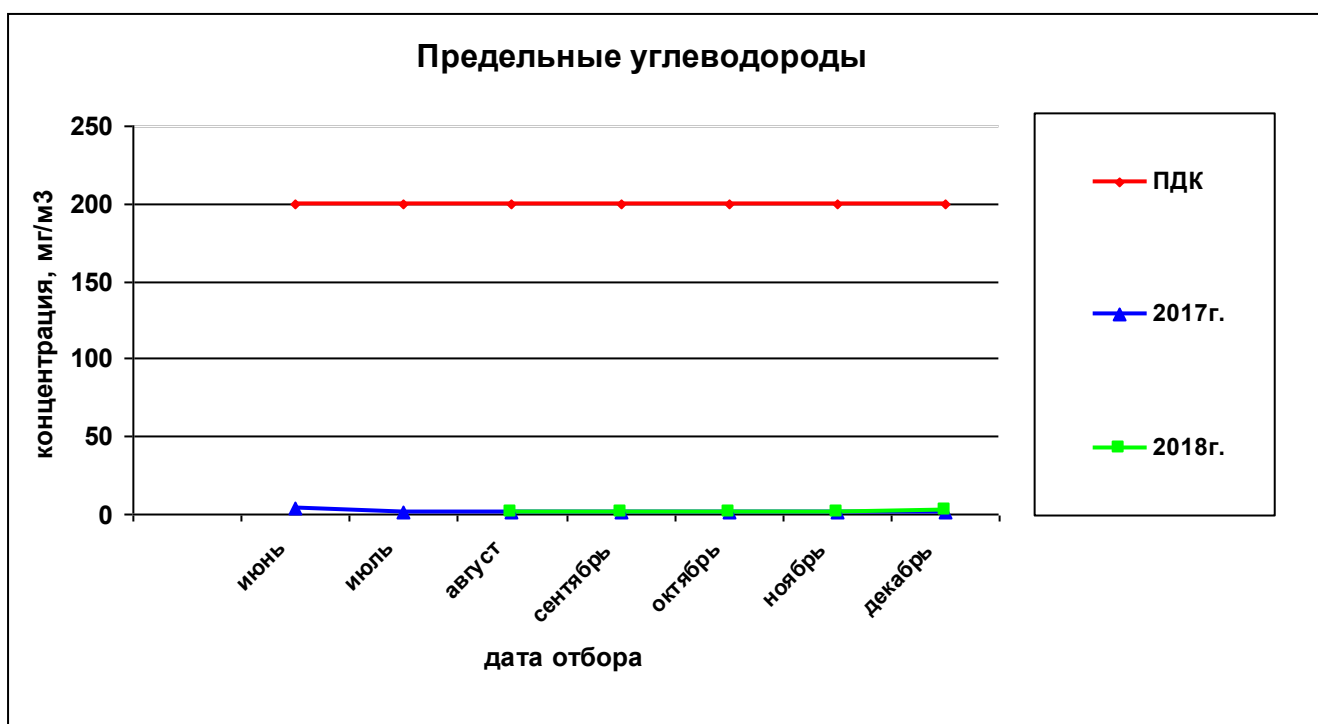
Рисунок 76— Сравнительная характеристика изменения концентрации предельных углеводородов в атмосферном воздухе на ул.Петропавловская,185 за 2017 и 2018гг.
