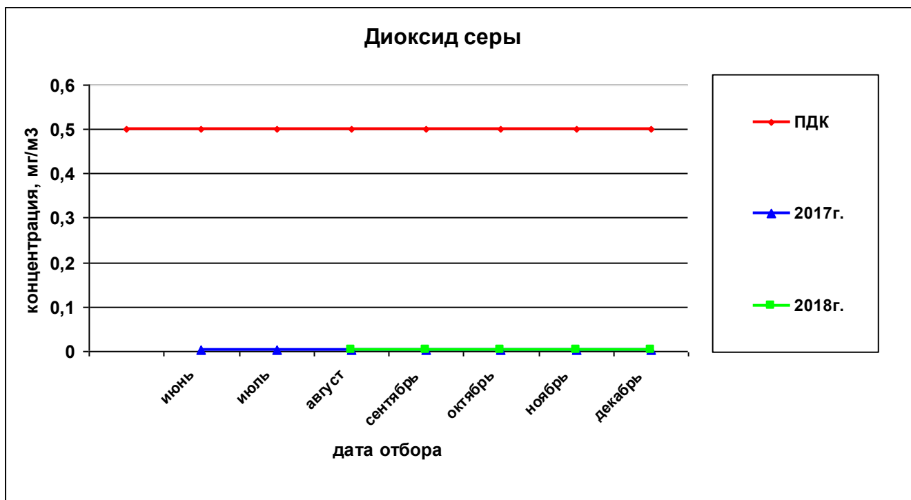
Рисунок 36— Сравнительная характеристика изменения концентрации диоксида серы в атмосферном воздухе на ул. Строителей за 2017 и 2018гг.
