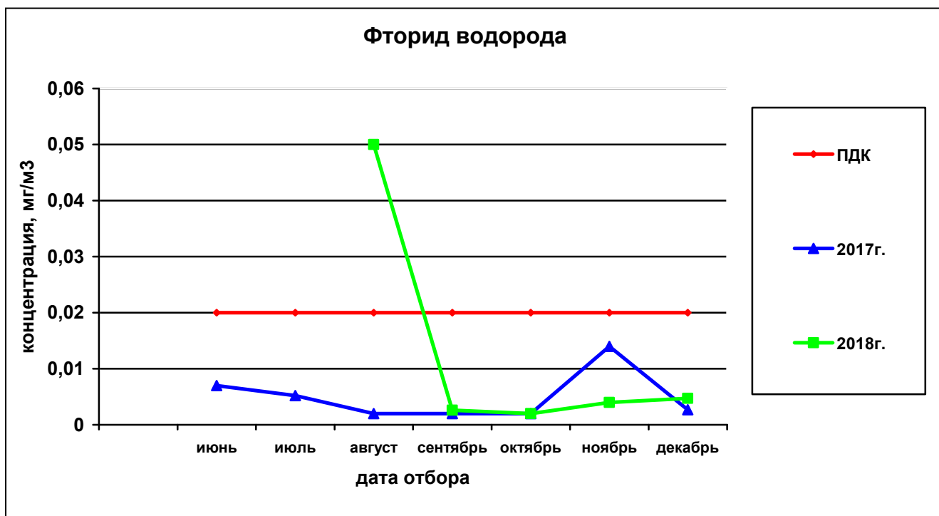
Рисунок 27— Сравнительная характеристика изменения концентрации фторида водорода в атмосферном воздухе на ул. Костычева за 2017 и 2018гг.
