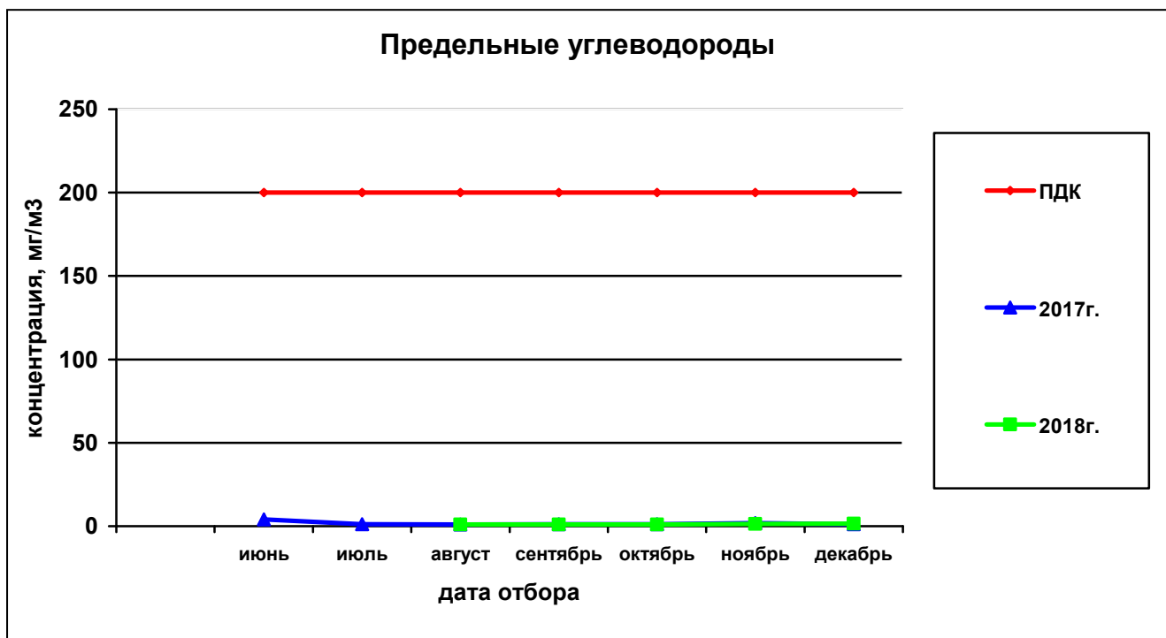
Рисунок 28— Сравнительная характеристика изменения концентрации предельных углеводородов в атмосферном воздухе на ул. Костычева за 2017 и 2018гг.
