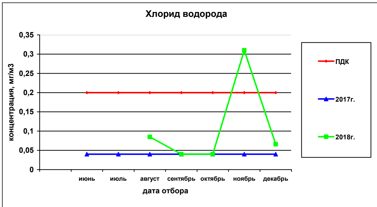
Рисунок 67— Сравнительная характеристика изменения концентрации хлорида водорода в атмосферном воздухе на ул.Петропавловская,185 за 2017 и 2018гг.
