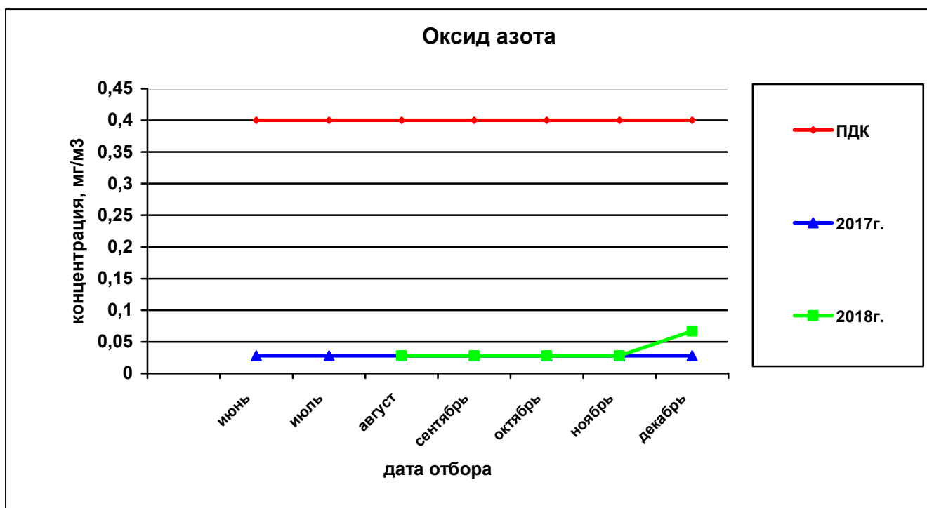
Рисунок 50— Сравнительная характеристика изменения концентрации оксида азота в атмосферном воздухе у домов по ул. Вавилова, 21 – Малкова, 22 за 2017 и 2018гг.
