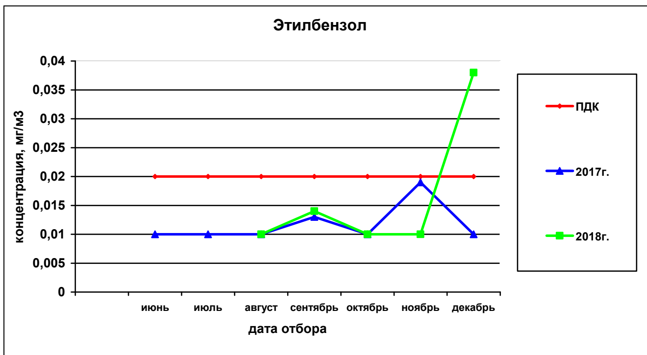
Рисунок 80— Сравнительная характеристика изменения концентрации этилбензола в атмосферном воздухе на ул.Петропавловская,185 за 2017 и 2018гг.
