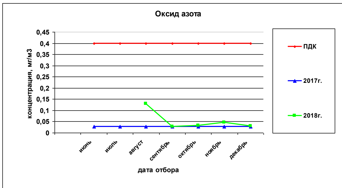
Рисунок 66— Сравнительная характеристика изменения концентрации оксида азота в атмосферном воздухе на ул.Петропавловская,185 за 2017 и 2018гг.
