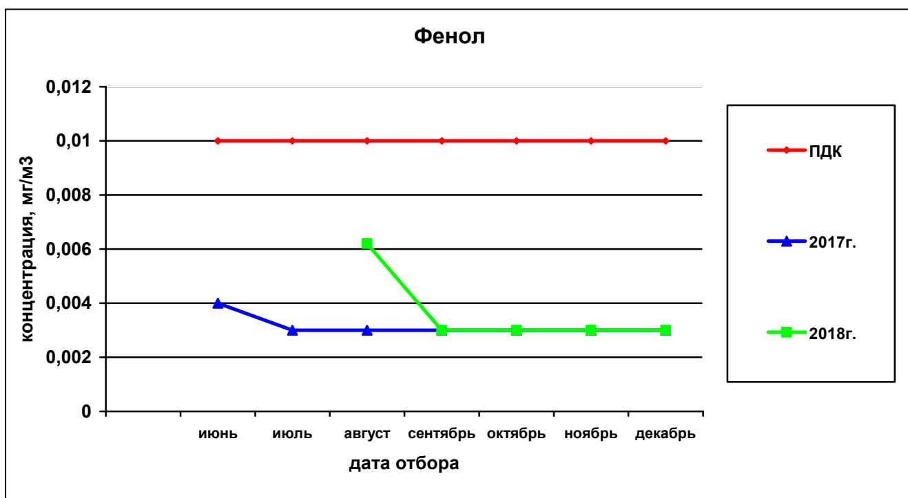
Рисунок 56— Сравнительная характеристика изменения концентрации фенола в атмосферном воздухе у домов по ул. Вавилова, 21 – Малкова, 22 за 2017 и 2018гг.
