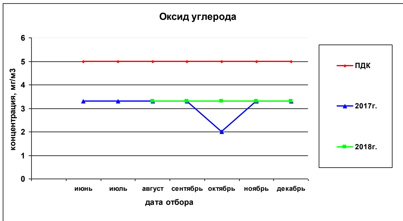
Рисунок 23— Сравнительная характеристика изменения концентрации оксида углерода в атмосферном воздухе на ул. Костычева за 2017 и 2018гг.
