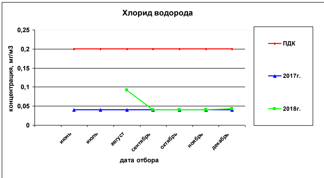
Рисунок 51— Сравнительная характеристика изменения концентрации хлорида водорода в атмосферном воздухе у домов по ул. Вавилова, 21 – Малкова, 22 за 2017 и 2018гг.
