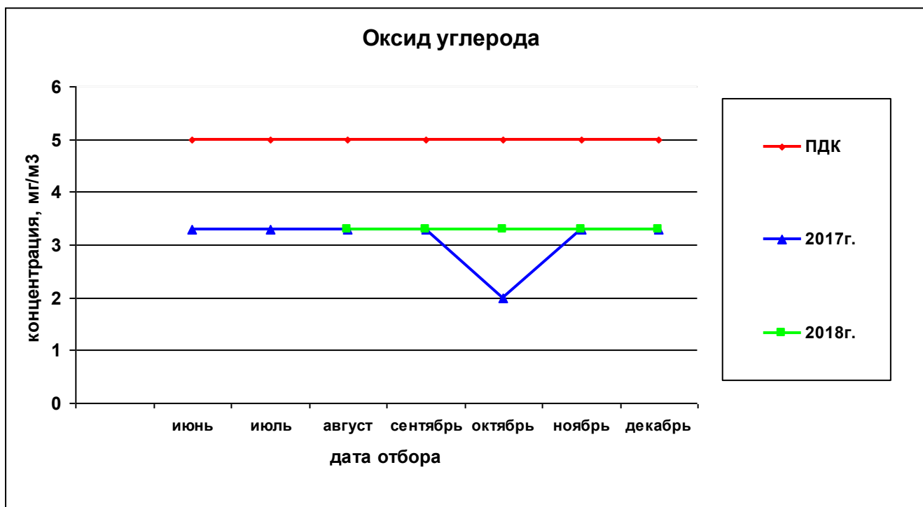
Рисунок 55— Сравнительная характеристика изменения концентрации оксида углерода в атмосферном воздухе у домов по ул. Вавилова, 21 – Малкова, 22 за 2017 и 2018гг.
