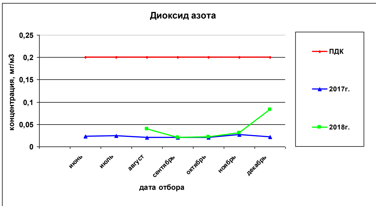
Рисунок 49— Сравнительная характеристика изменения концентрации диоксида азота в атмосферном воздухе у домов по ул. Вавилова, 21 – Малкова, 22 за 2017 и 2018гг.
