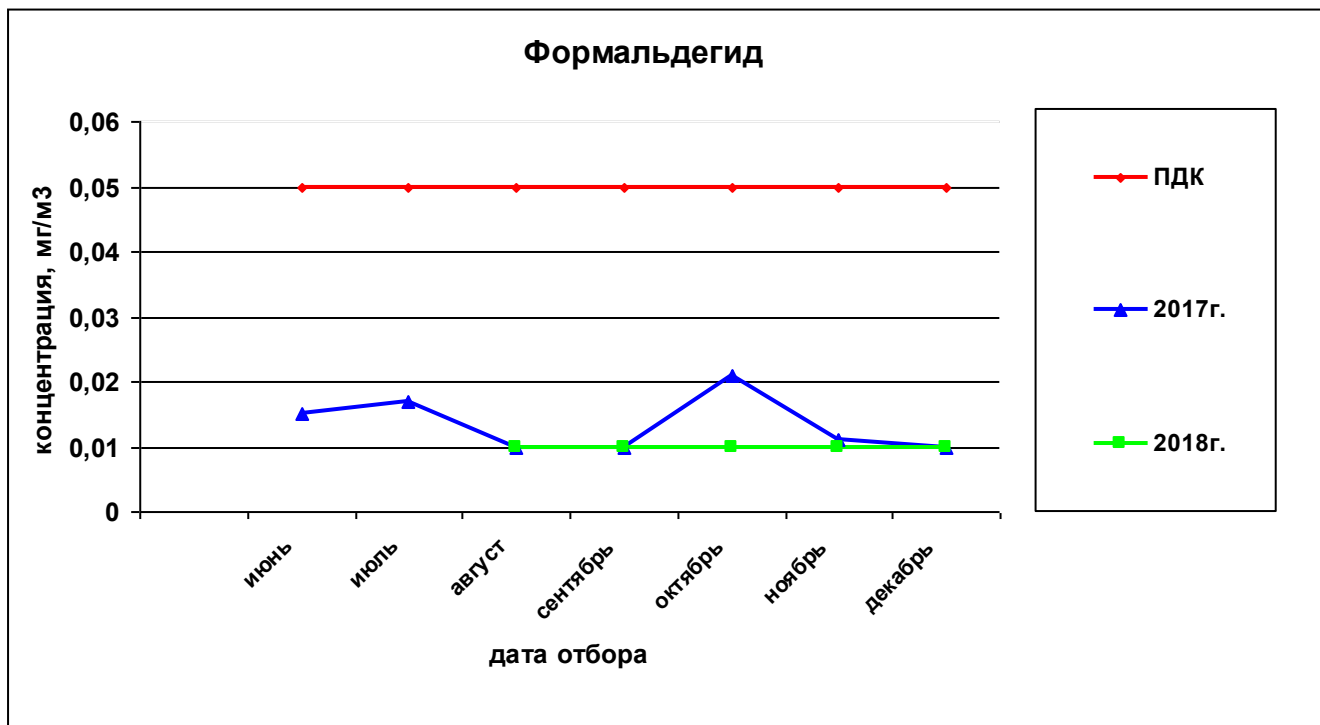
Рисунок 57— Сравнительная характеристика изменения концентрации формальдегида в атмосферном воздухе у домов по ул. Вавилова, 21 – Малкова, 22 за 2017 и 2018гг.
