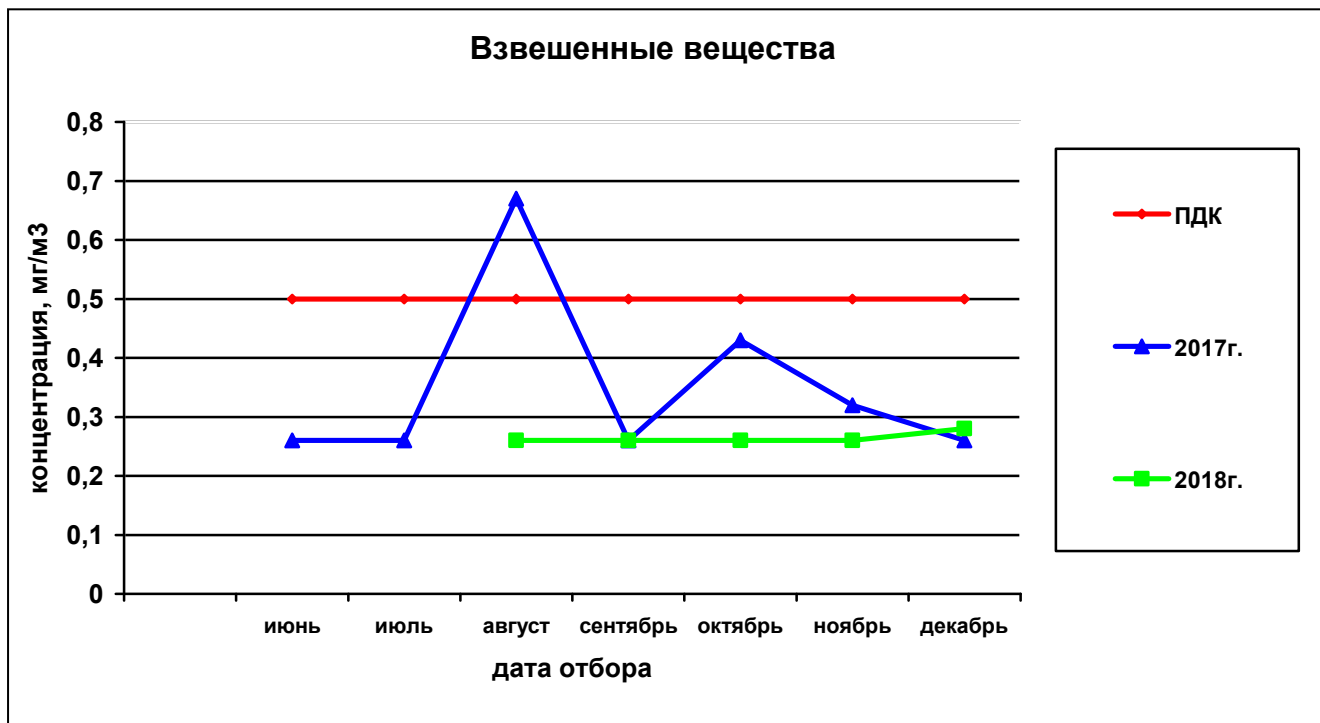
Рисунок 58— Сравнительная характеристика изменения концентрации взвешенных веществ в атмосферном воздухе у домов по ул. Вавилова, 21 – Малкова, 22 за 2017 и 2018гг.
