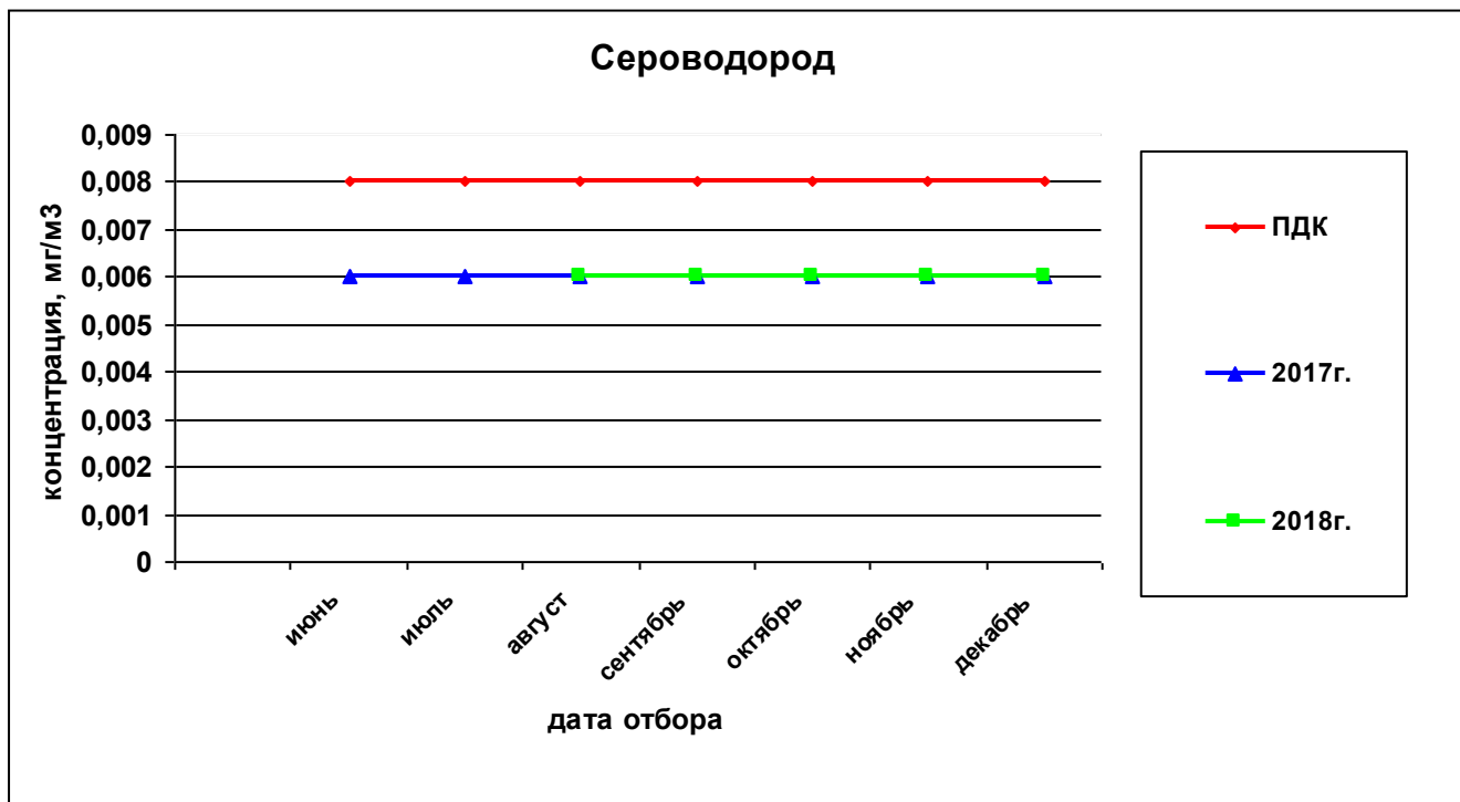
Рисунок 69— Сравнительная характеристика изменения концентрации сероводорода в атмосферном воздухе на ул.Петропавловская,185 за 2017 и 2018гг.
