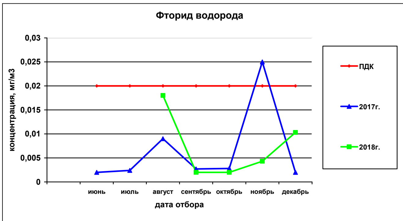
Рисунок 59— Сравнительная характеристика изменения концентрации фторида водорода в атмосферном воздухе у домов по ул. Вавилова, 21 – Малкова, 22 за 2017 и 2018гг.
