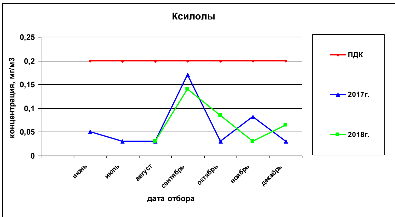
Рисунок 79— Сравнительная характеристика изменения концентрации ксилолов в атмосферном воздухе на ул.Петропавловская,185 за 2017 и 2018гг.
