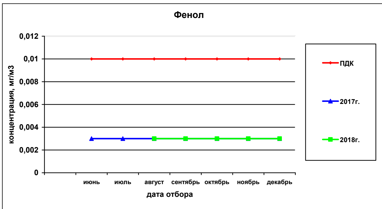
Рисунок 40— Сравнительная характеристика изменения концентрации фенола в атмосферном воздухе на ул. Строителей за 2017 и 2018гг.
