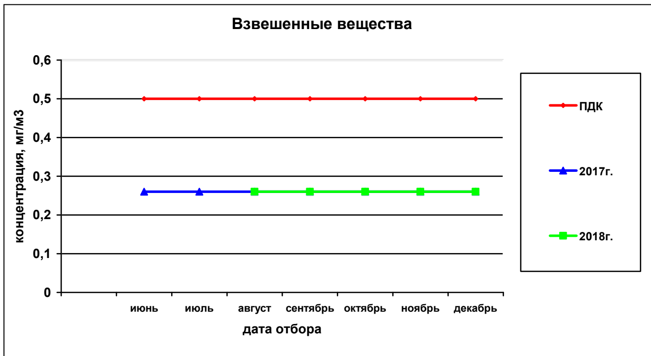
Рисунок 26— Сравнительная характеристика изменения концентрации взвешенных веществ в атмосферном воздухе на ул. Костычева за 2017 и 2018гг.
