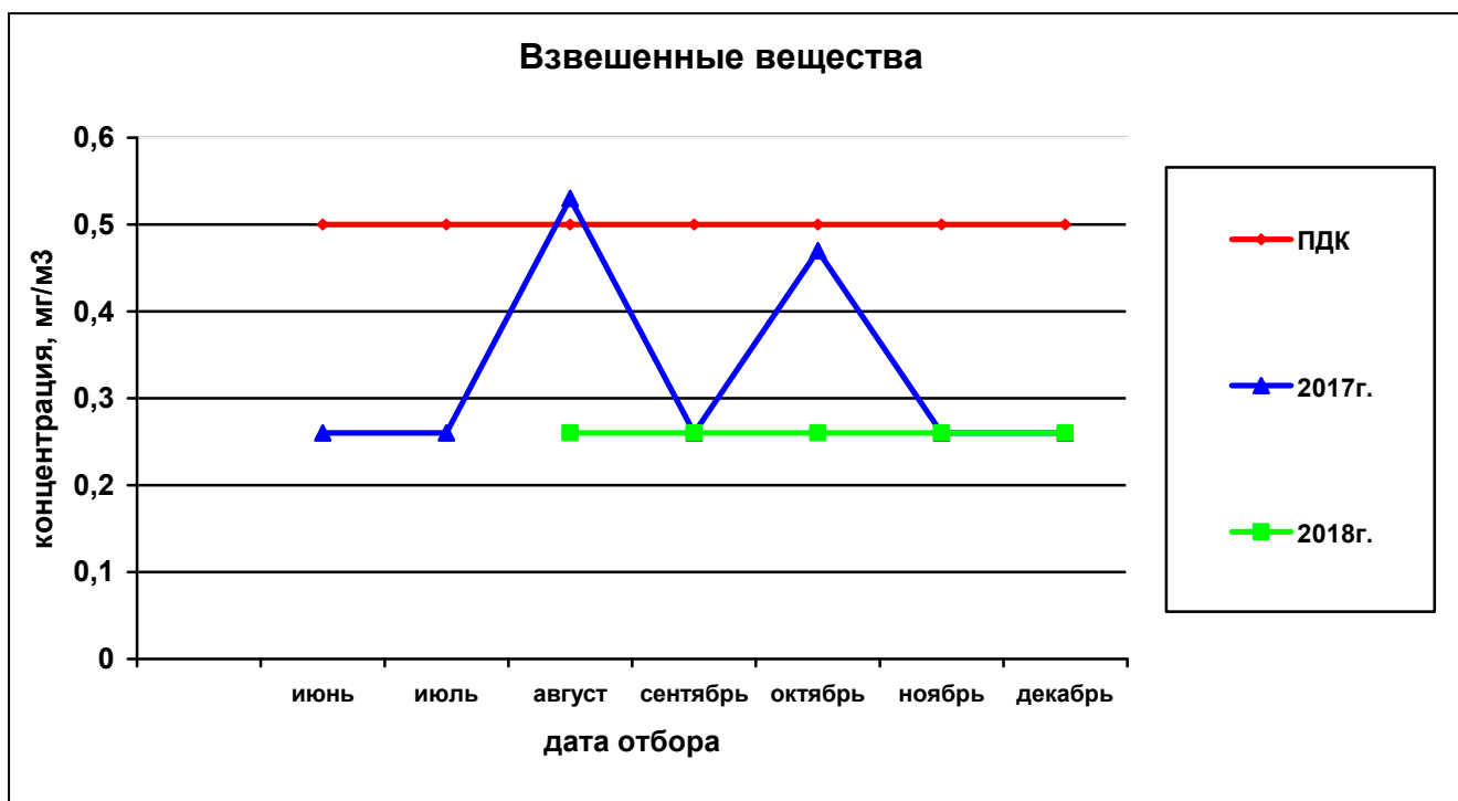
Рисунок 74— Сравнительная характеристика изменения концентрации взвешенных веществ в атмосферном воздухе на ул.Петропавловская,185 за 2017 и 2018гг.
